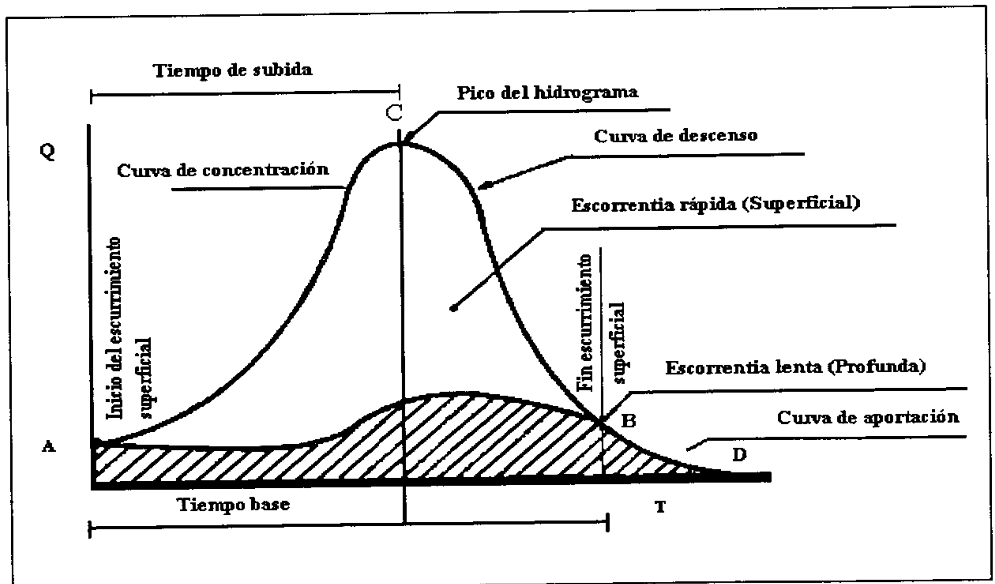
Figura 1: Componentes del hidrograma (TRAGSA, 1994).
