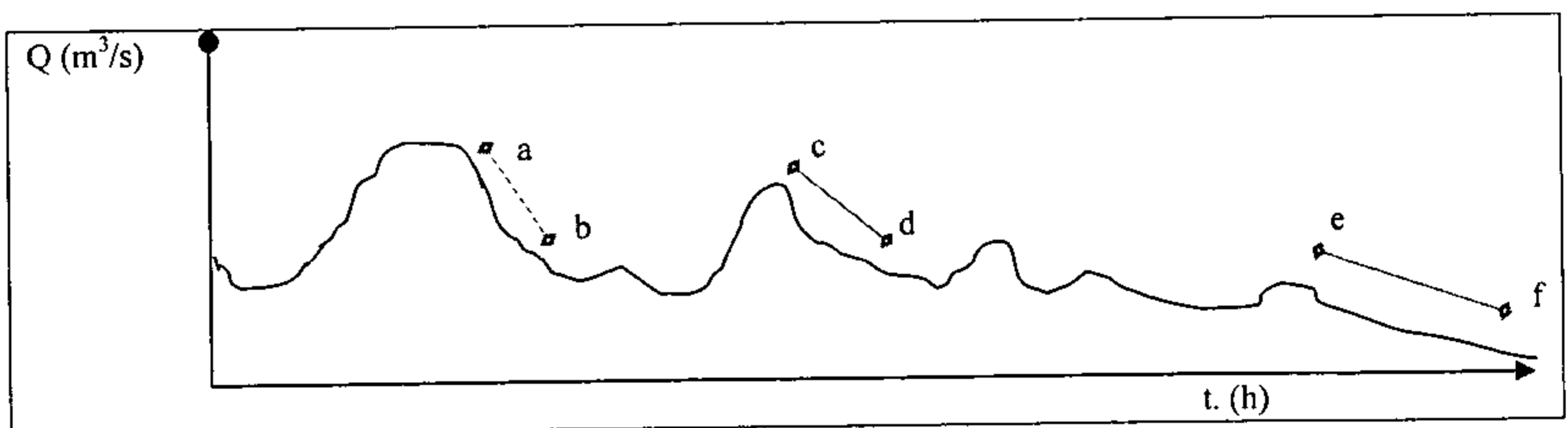
Figura 2: Hidrograma de escurrientías superficial y subterránea.
