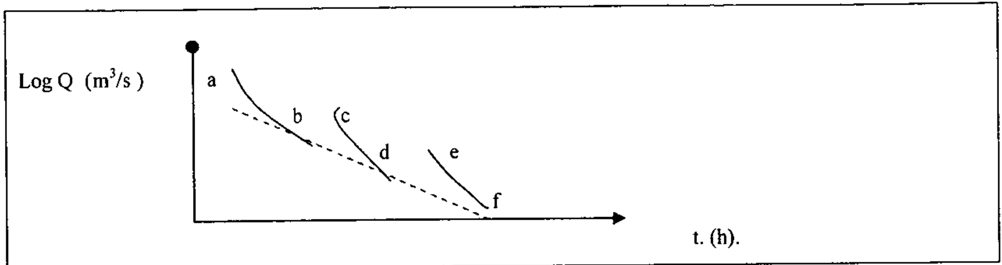
Figura 3: Curva de vaciado del gasto base.
