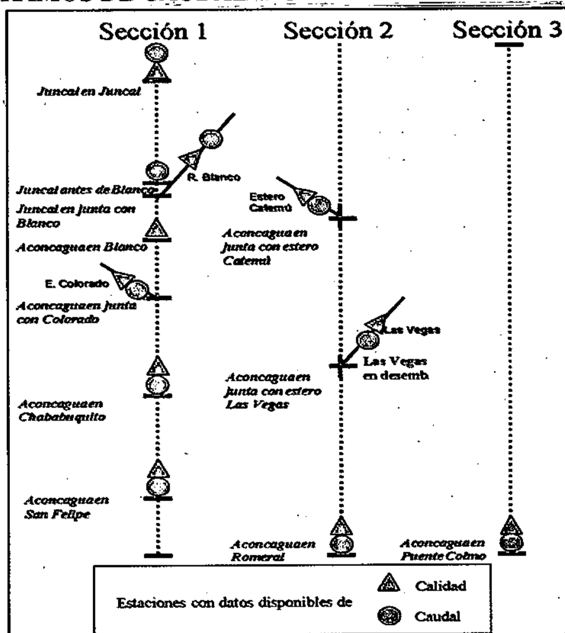
FIGURA 9 DIAGRAMA DE DIVISIÓN DEL RÍO EN SECCIONES Y TRAMOS DE CAUDAL Y CALIDAD HOMOGÉNEOS
