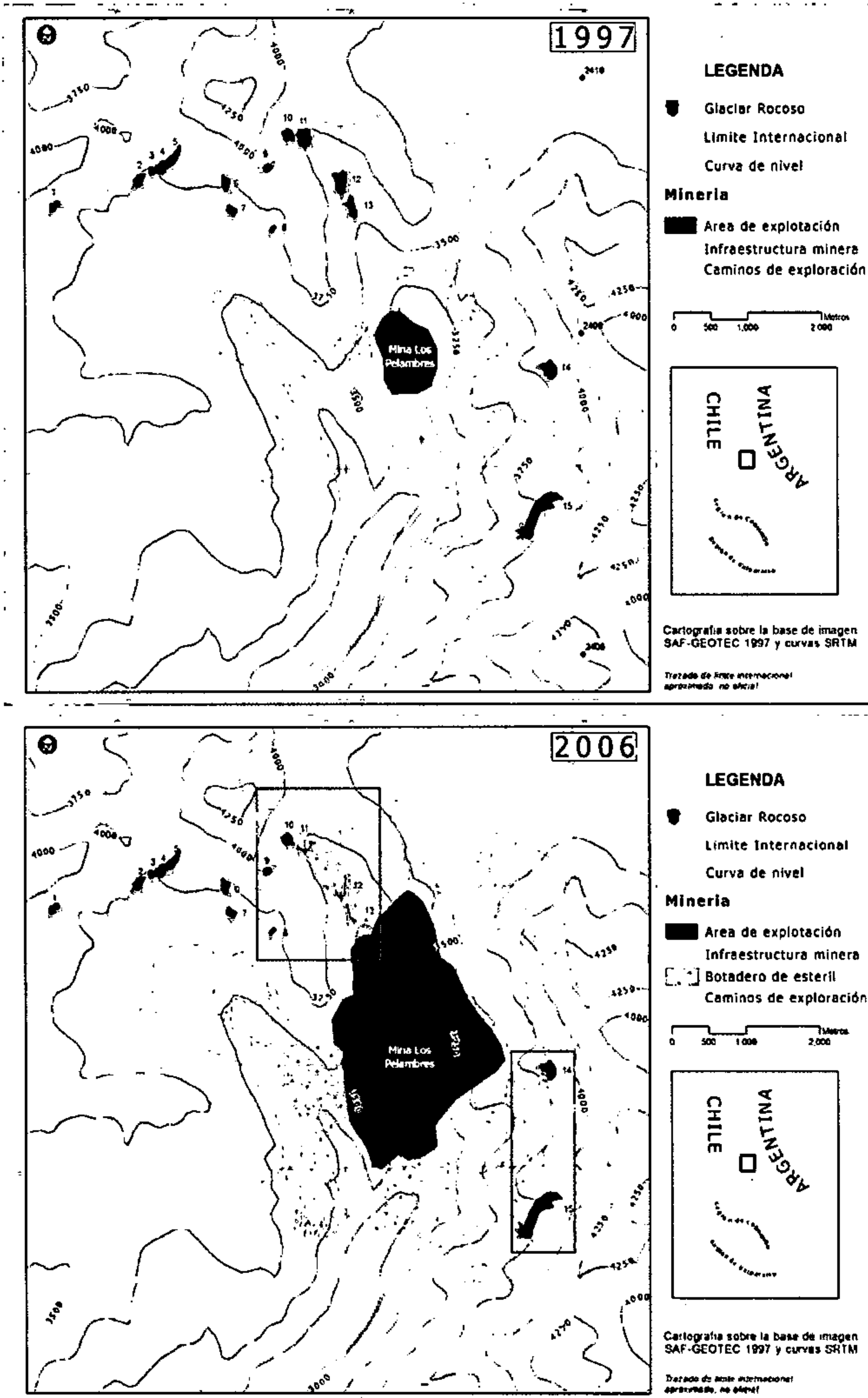
Figura N° 1: Glaciares rocosos afectados por Minera Los Pelambres entre los años 1997 y 2006.
