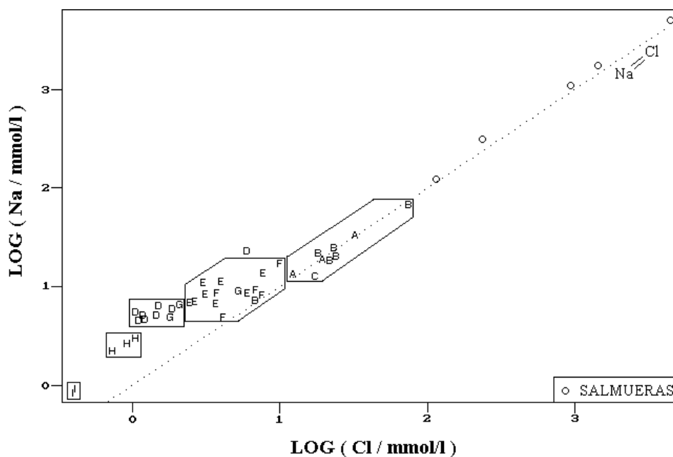
Fig. 4. Relación Na versus Cl en las aguas y salmueras de Pintados.
