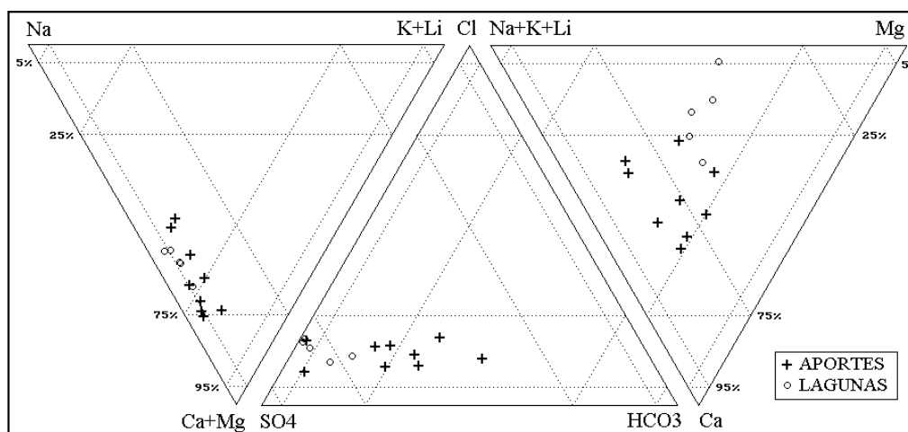
Fig.1. Composición de las aguas de aporte y de salmueras del salar de Michincha.
