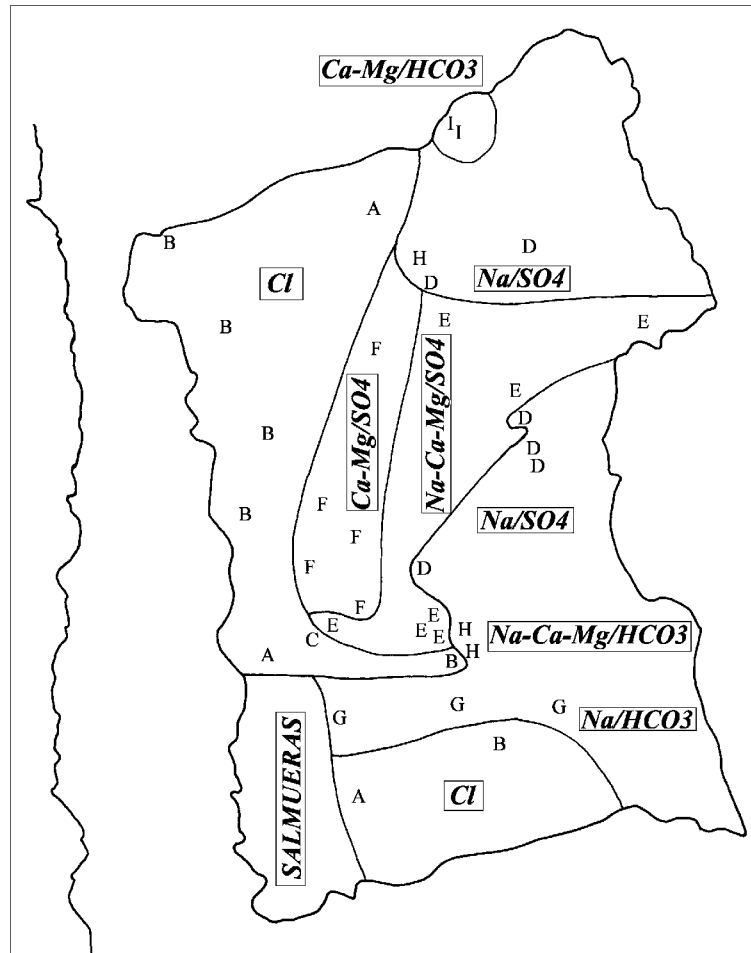
Fig.3 : Distribución geográfica de los varios tipos de agua en el salar de Pintados. La letras corresponden a los tipos químicos definidos en la figura 2.
