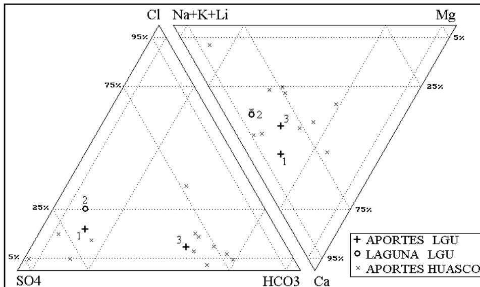
Fig.1 : Composición química de las aguas de Lagunilla y de los aportes al salar del Huasco.
