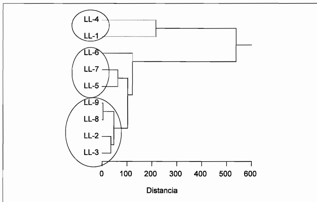
Figura 12. Análisis de conglomerados. Segregación espacial de las estaciones de muestreo en función de la densidad total y riqueza de taxa de macroinvertebrados bentónicos. Estudio de limnología. Río Lluta. Diciembre de 2008.
