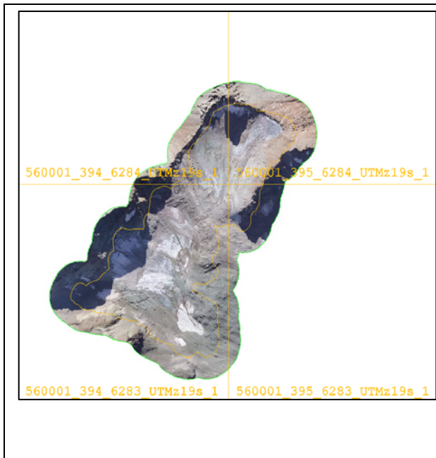
Figura 15: Imágenes ortorectificadas.
