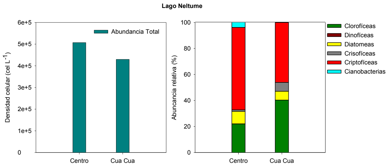
Fig. 11 a) Densidad celular y b) abundancia relativa de microalgas registradas en las estaciones de muestro pelágico del lago Neltume, estaciones Centro y Cua-Cua.
