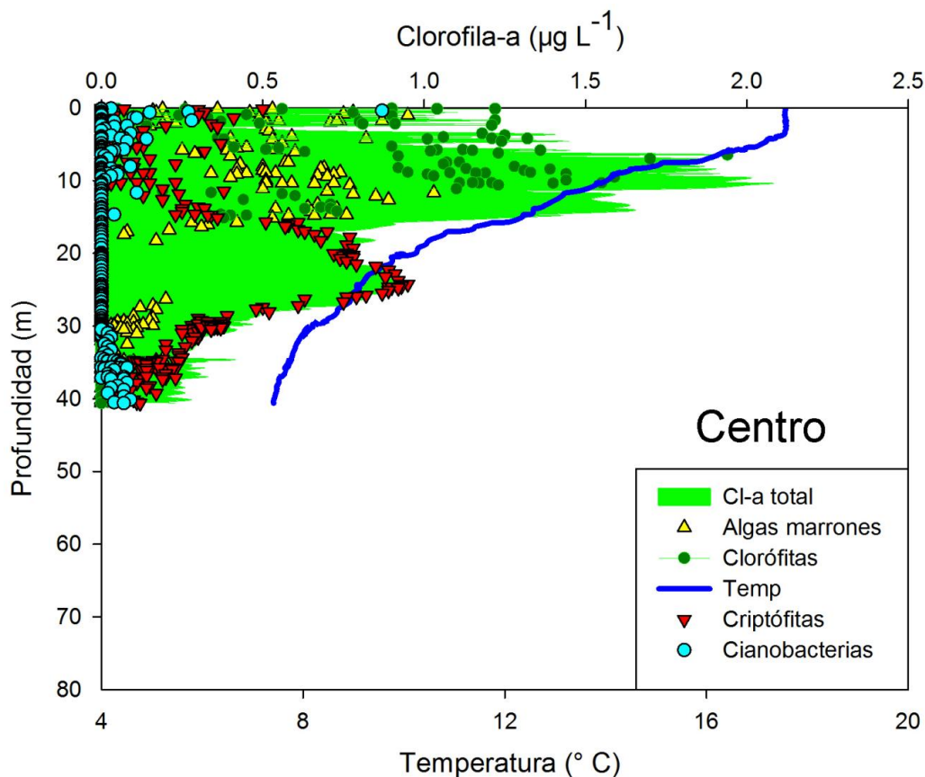
Fig. 7 Distribución vertical de la clorofila-a “total” (área verde) y la biomasa proporcional para las Clorófitas (círculos verdes), Cianobacterias (círculos azules), Criptofíceas (triángulos rojos) y algas marrones (Diatomeas, Crisofíceas y Dinofíceas; triángulos amarillos) en la estación Centro del lago Neltume.
