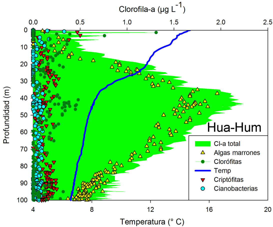
Fig. 21 Distribución vertical de la clorofila-a “total” (área verde) y la biomasa proporcional para las Clorófitas (círculos verdes), Cianobacterias (círculos azules), Criptófitas (triángulos rojos) y algas marrones (Diatomeas, Crisófitas y Dinófitas; triángulos amarillos) en la estación Hua-Hum del lago Pirehueico.
