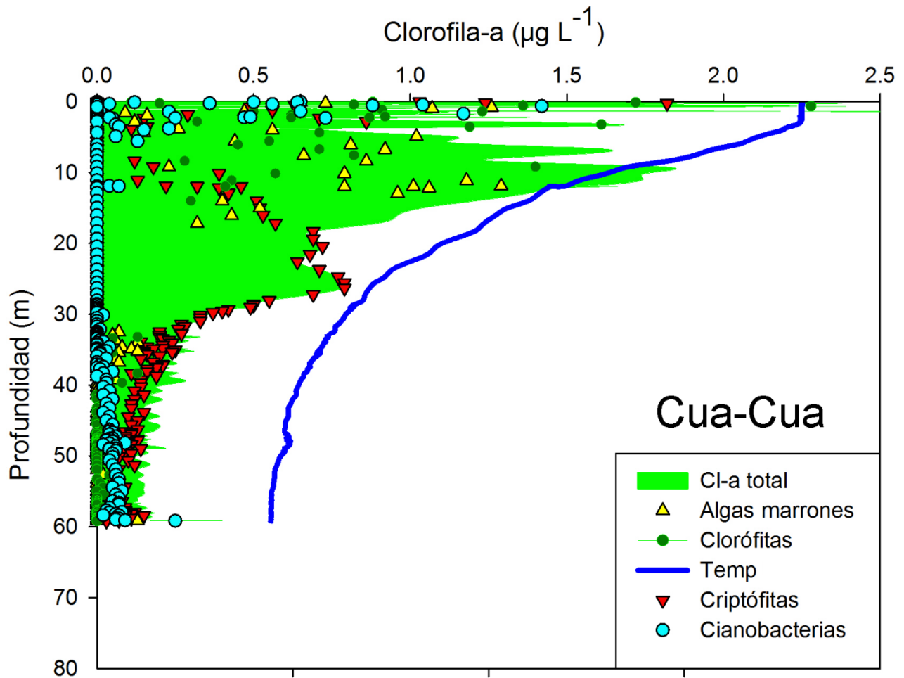
Fig. 9 Distribución vertical de la clorofila-a “total” (área verde) y la biomasa proporcional para las Clorófitas (círculos verdes), Cianobacterias (círculos azules), Criptófitas (triángulos rojos) y algas marrones (Diatomeas, Crisofíceas y Dinofíceas; triángulos amarillos) en la estación Cua-Cua.
