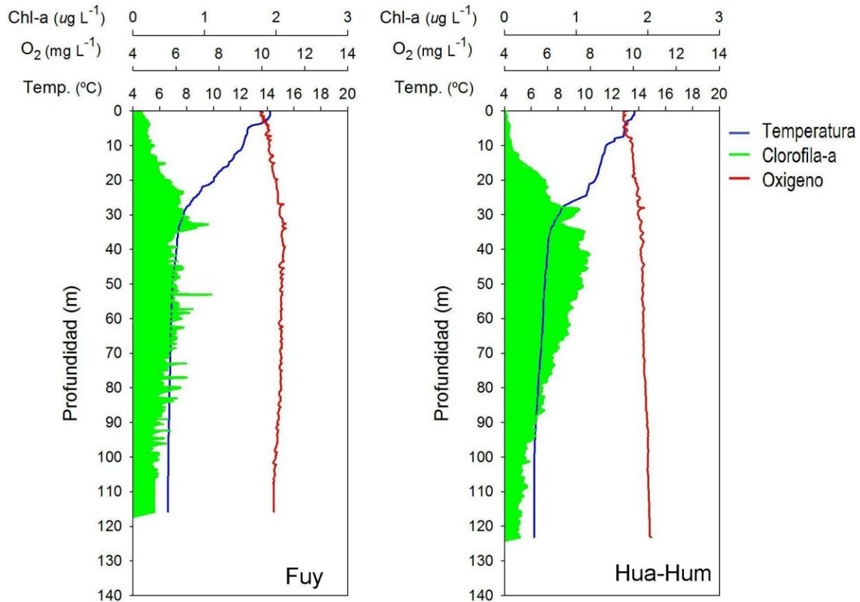
Fig. 16 Perfiles verticales de la temperatura, oxígeno disuelto y clorofila-a medidos en el lago Pirehueico
