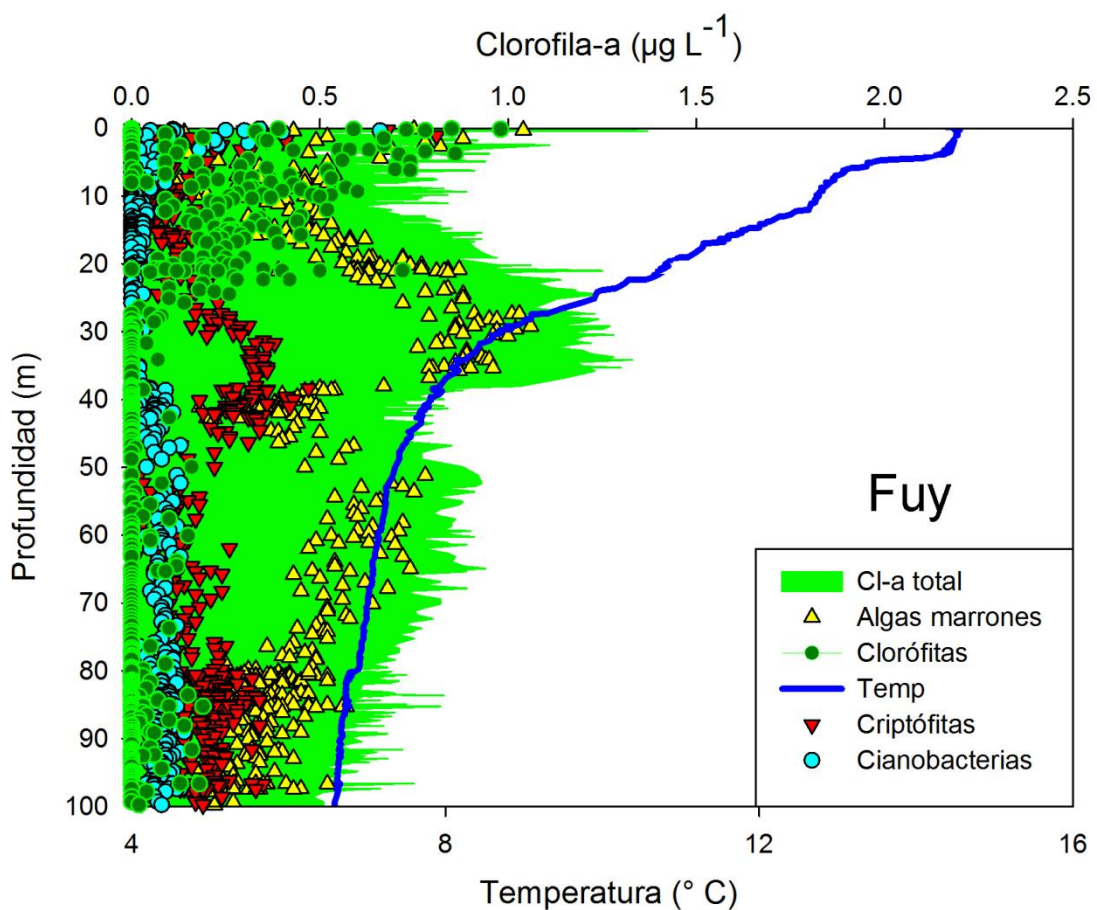
Fig. 19 Distribución vertical de la clorofila-a “total” (área verde) y la biomasa proporcional para las Clorofíceas (círculos verdes), Cianobacterias (círculos azules), Criptofíceas (triángulos rojos) y algas marrones (Diatomeas, Crisofíceas y Dinofíceas; triángulos amarillos) en la estación Fuy del lago Pirehueico.
