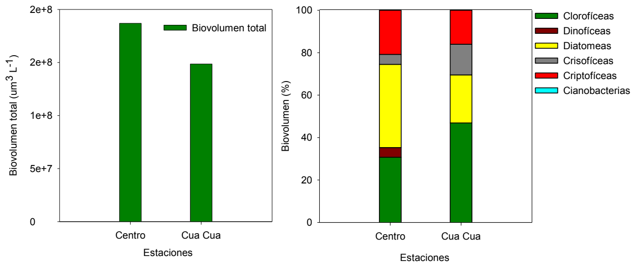
Fig. 12. a) Biovolumen de fitoplancton y b) biomasa (biovolumen) relativo de microalgas registradas en las estaciones de muestro pelágico del lago Neltume, estaciones Centro y Cua-Cua.
