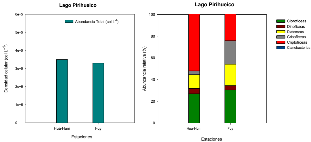
Fig.23 a) Densidad celular y b) abundancia relativa de microalgas registradas en las estaciones de muestro pelágico del lago Pirehueico, estaciones Hua-Hum y Fuy.
