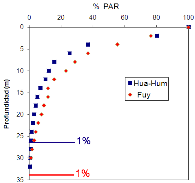
Fig. 18 Perfil vertical de la luz visible (PAR: 400-700 nm) y la zona eufótica (1%) en las estaciones Hua-Hum y Fuy.
