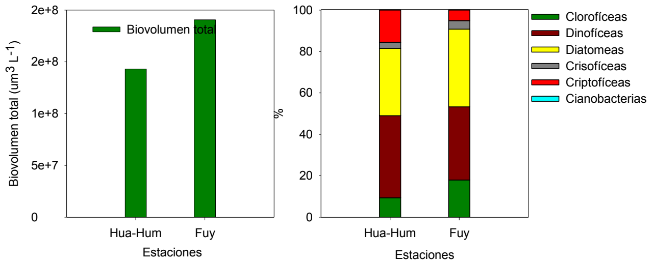
Fig.24. a) Biovolumen de fitoplancton y b) biomasa (bio-volumen) relativa de microalgas registradas en las estaciones de muestro pelágico del lago Pirehueico, estaciones Hua-Hum y Fuy.
