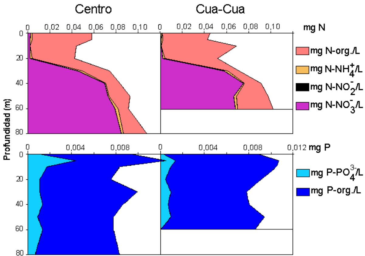
Fig. 5 Perfiles verticales de diferentes fracciones de nitrógeno y fósforo en dos estaciones en el lago Neltume. N-org. = nitrógeno orgánico. P-org. = fósforo orgánico. Valores son acumulativos. La suma de los valores corresponde a P total y N total.
