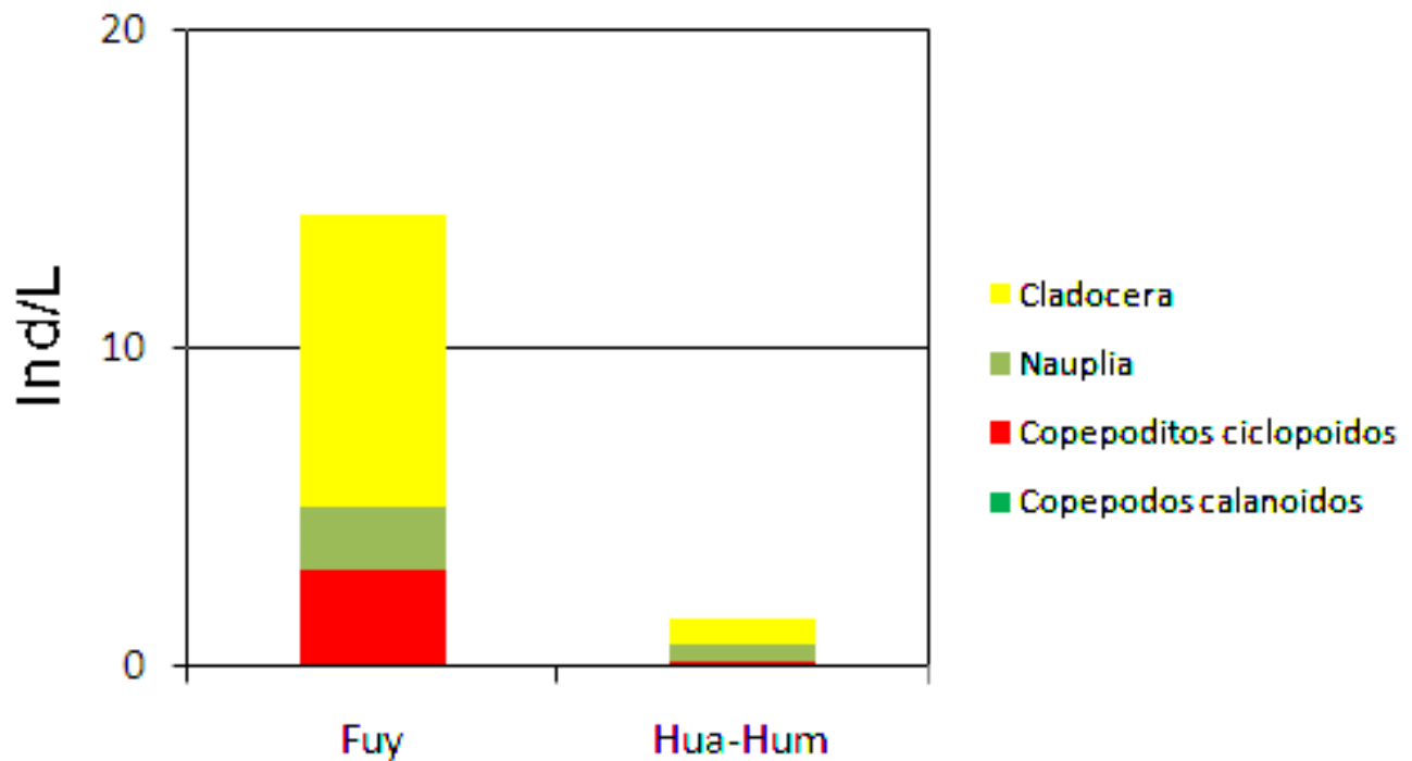
Fig.25 Abundancia de los grupos de microcrustáceos en dos estaciones del lago Neltume
