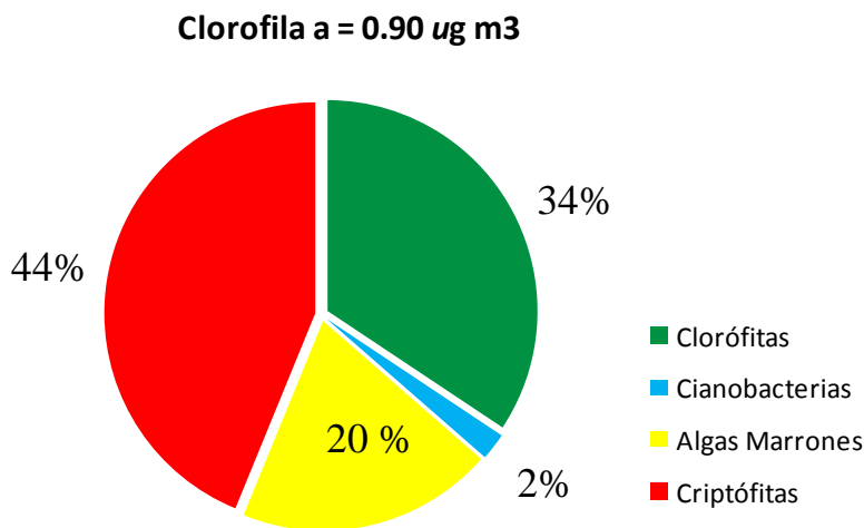
Fig. 8 Valor medio integrado de clorofila-a, 0-40m, en la estación Centro del lago Neltume y biomasa proporcional para los distintos grupos de microalgas.
