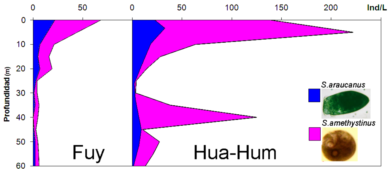
Fig. 26 Distribución vertical de Stentor araucanus (azul) y Stentor amethystinus (rosado) en dos estaciones en el lago Pirehueico (15.11.2012)
