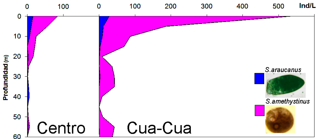
Fig. 15 Distribución vertical de Stentor araucanus (azul) y Stentor amethystinus (rosa) en dos estaciones en el lago Neltume (16.11.2012)
