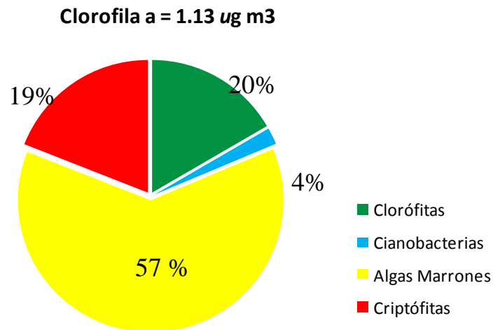
Fig. 22 Valor medio integrado de clorofila, 0-40m, en la estación Hua-Hum del lago Pirehueico y biomasa proporcional de cl-a para los distintos grupos de microalgas.
