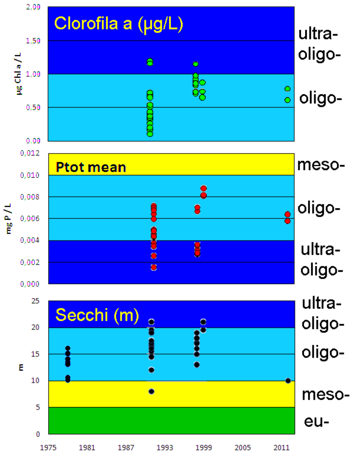
Fig. 28 Estado trófico del lago Pirehueico, basado en la transparencia y promedio de fósforo total (PT) (0-140 m) y de clorofila a (0-40 m) en estaciones pelágicas. Datos en Anexo 1.
