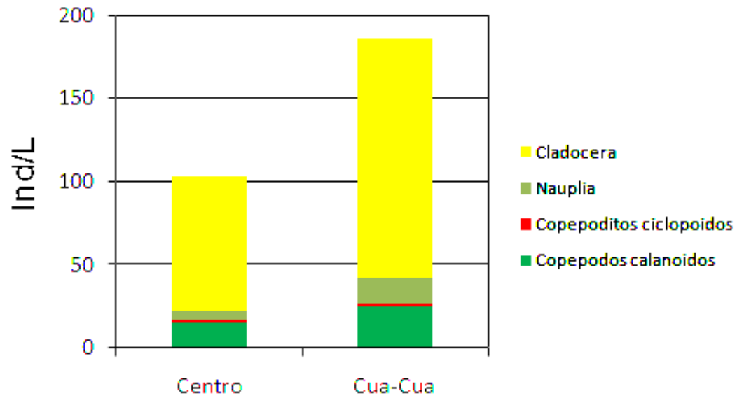
Fig. 13 Abundancia de los grupos de microcrustáceos en dos estaciones del lago Neltume
