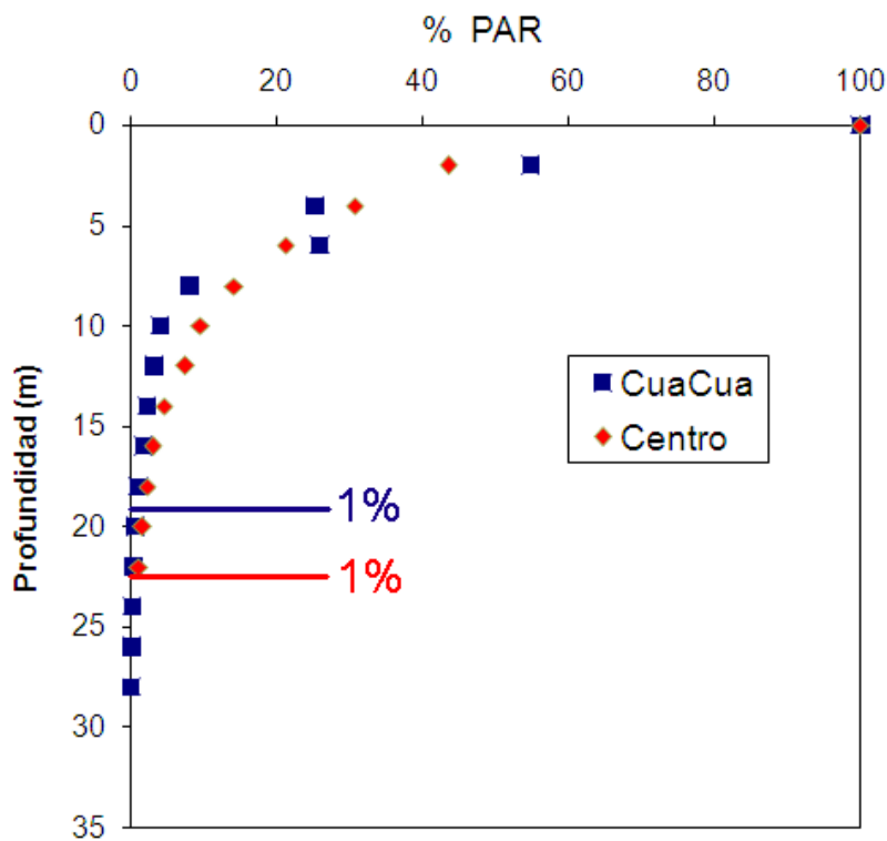
Fig. 6 Perfil vertical de atenuación la luz visible (PAR: 400-700 nm) y ubicación del límite inferior de la zona eufótica (1%) en las estaciones Centro y Cua-Cua
