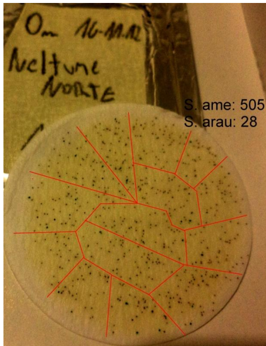
Fig. 3 Ciliados (puntos oscuros) sobre filtro de fibra de vidrio (0,7 \mu m). Tomado en estación Cua-Cua (Lago Neltume, superficie. Volumen filtrado: 1 L)
