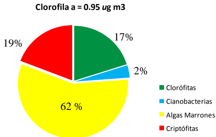
Fig. 20 Valor medio integrado de clorofila, 0-40m, en la estación Fuy del lago Pirehueico y biomasa proporcional de cl-a para los distintos grupos de microalgas.
