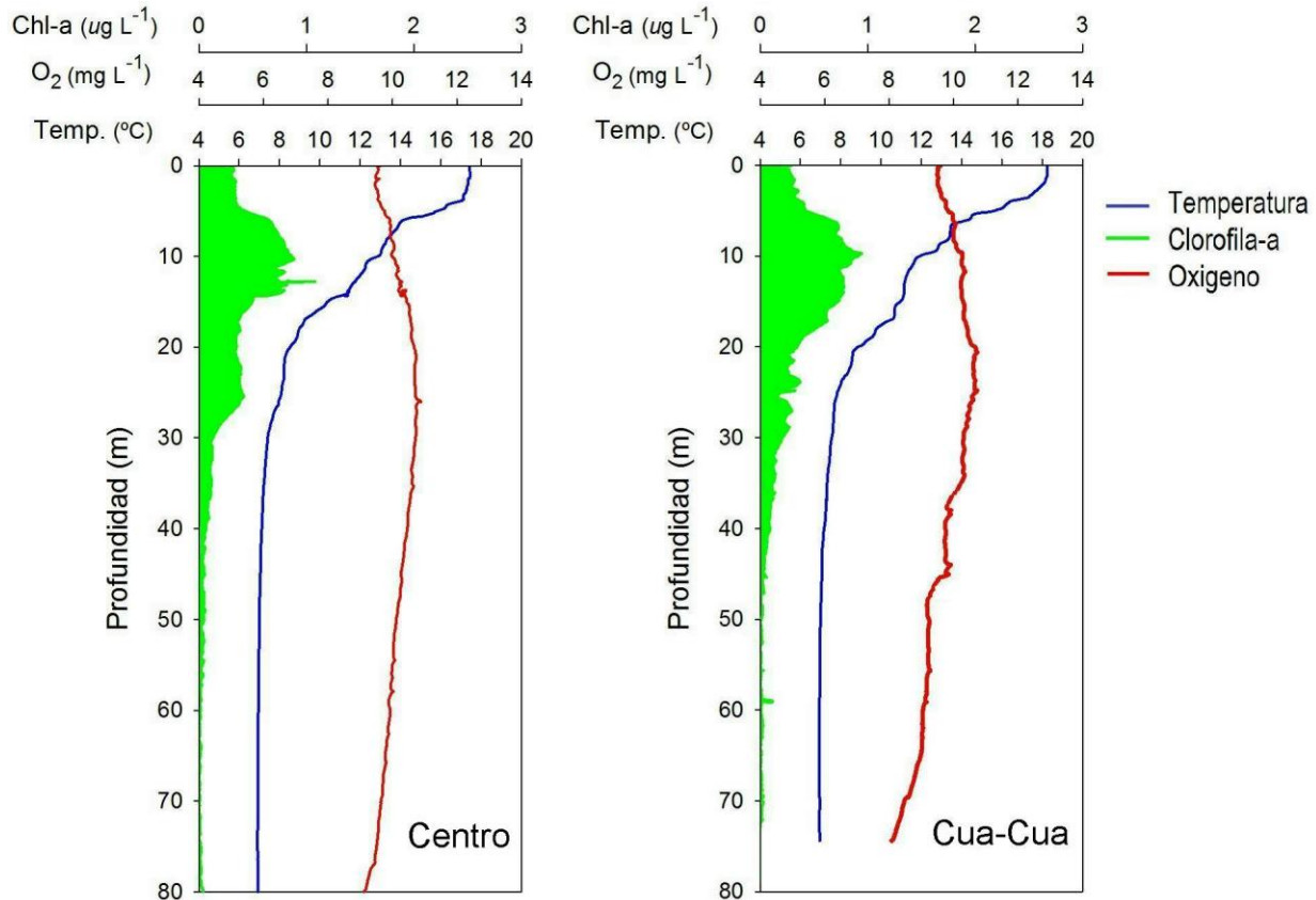
Fig. 4 Perfiles verticales de la temperatura (°C), oxígeno disuelto (mg/L) y clorofila-a (µg/L) medidos en el lago Neltume
