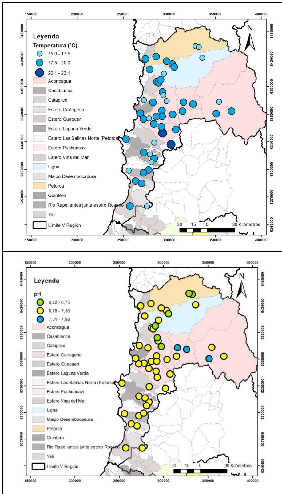
Figura 14: Parámetros físico químicos registrados in-situ en aguas de 49 pozos de la V Región. Arriba: datos de T; Abajo: datos de pH.
