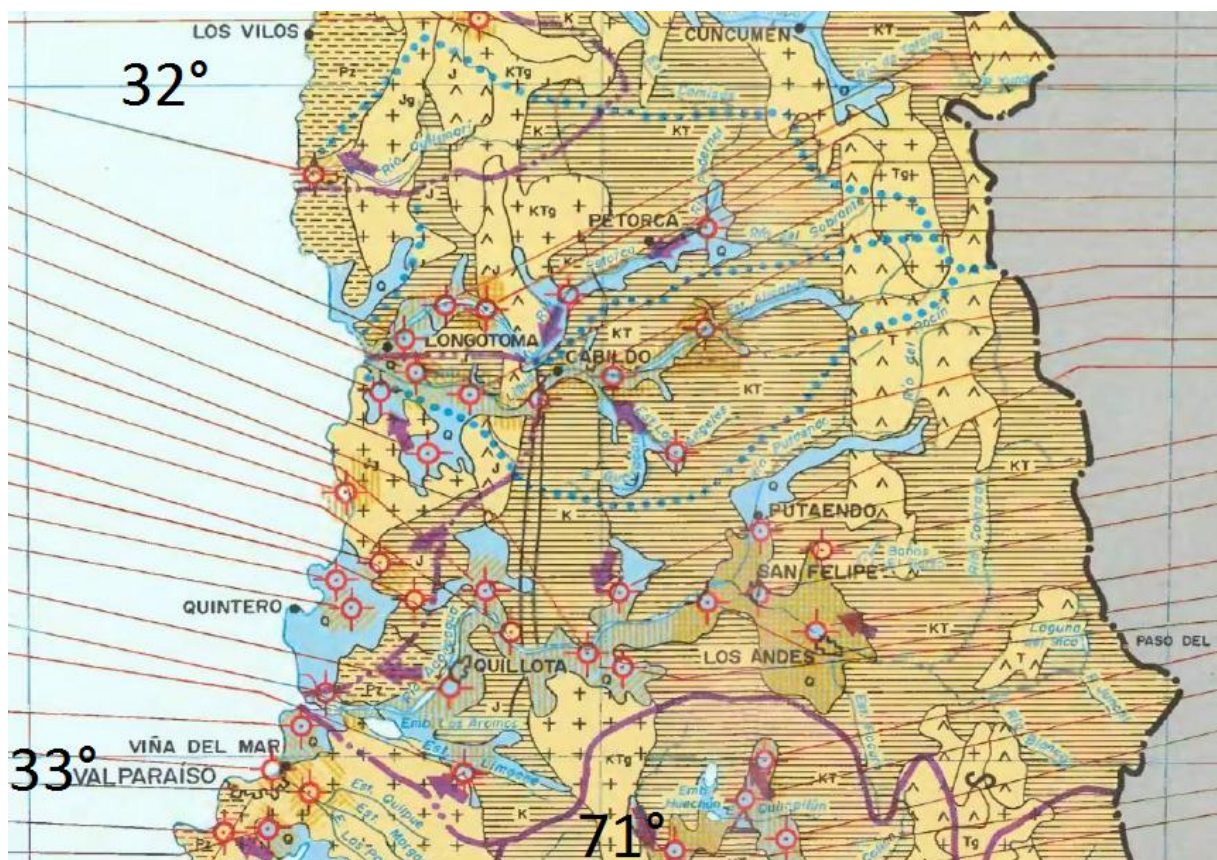
Figura 3: Extracto de Mapa hidrogeológico, DGA. Representa la V región. Para tener información más detallada de simbología se recomienda revisar la fuente.
