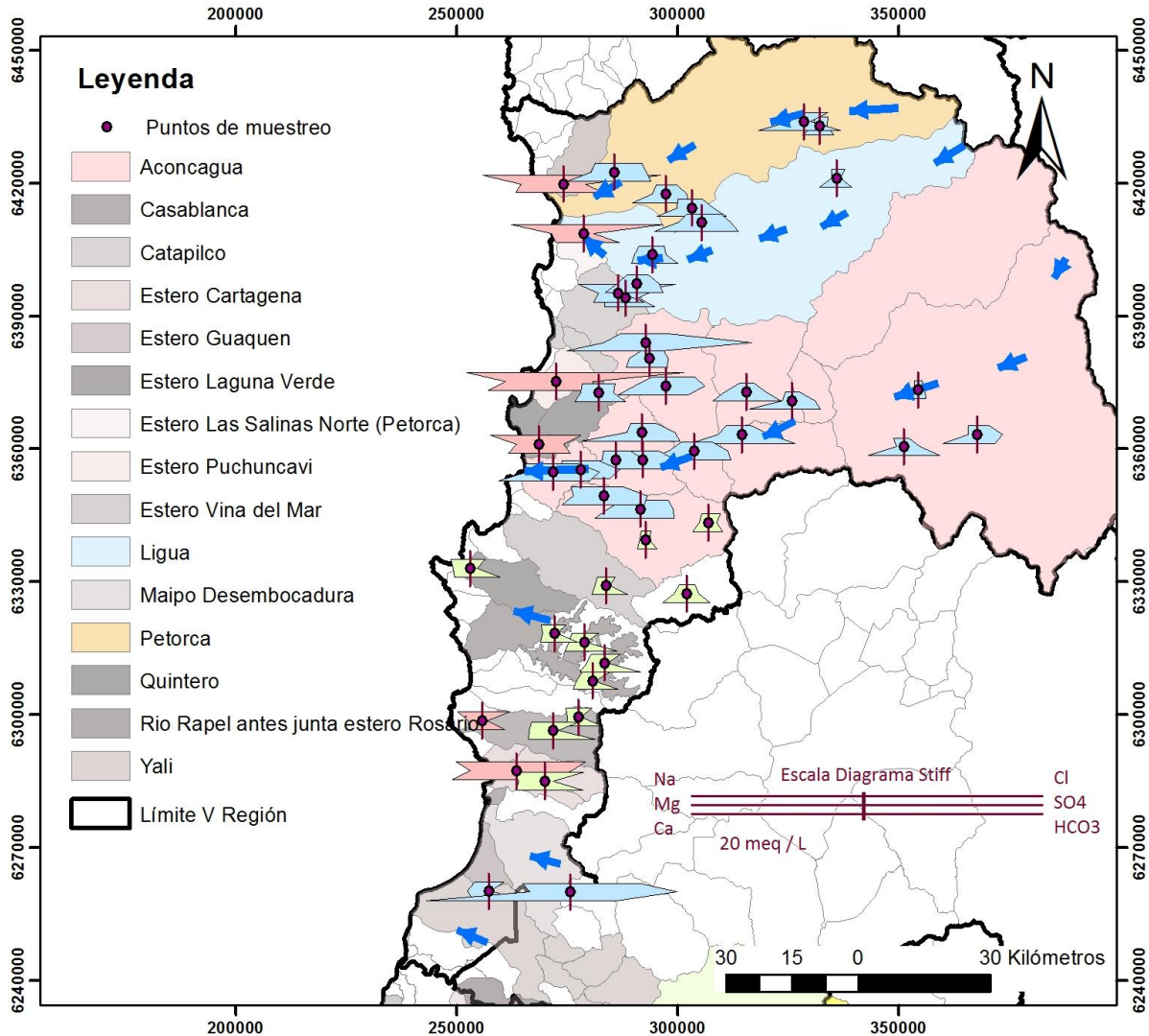
Figura 17: Diagramas de Stiff-modificado para las 49 muestras de aguas subterráneas tomadas en la V región. Los diagramas de aguas bicarbonatadas cálcicas se muestran en color celeste, los de aguas cloruradas sódicas en color rosado y las bicarbonatadas o cloruradas cálcicas en color verde.
