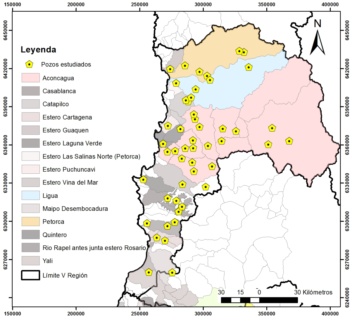
Figura 10: Distribución de puntos de muestreo.
