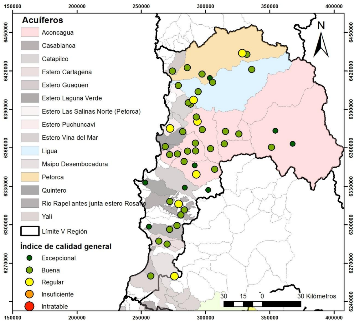
Figura 30: Resultados de Análisis de Índice de calidad de los pozos estudiados en la V Región.
