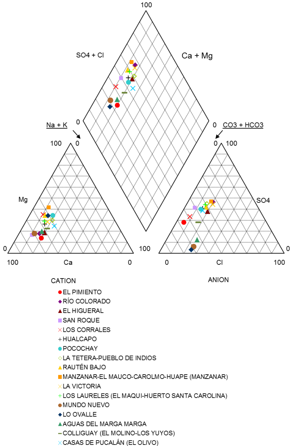
Figura 20: Representación mediante diagrama de Piper de las características químicas de las aguas subterráneas muestreadas en el acuífero Aconcagua. Se puede clasificar entre bicarbonatada o sulfatada cálcica. Lo que indicaría procesos que ocurren en rocas carbonatadas o cristalinas y procesos de reducción de yeso u oxidación de sulfatos.
