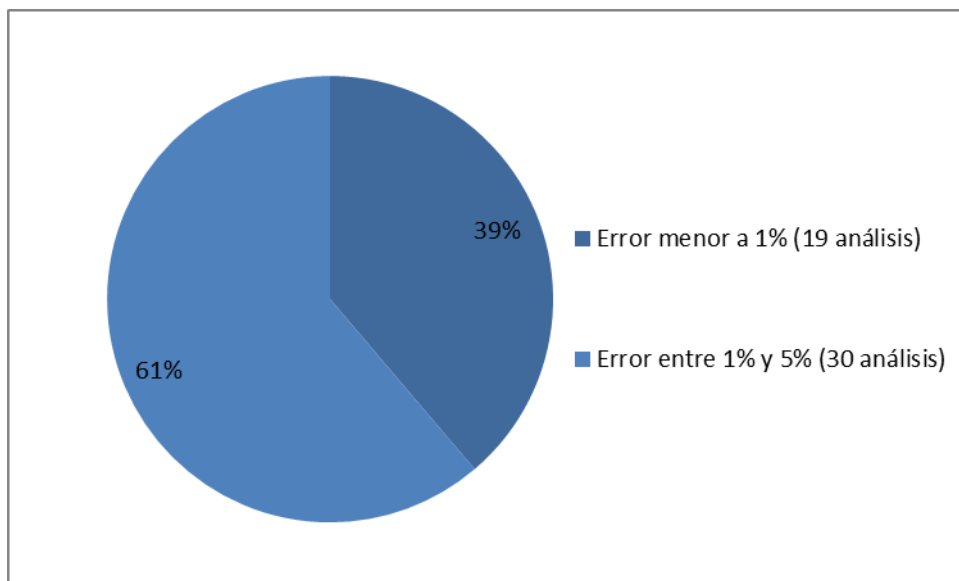
Figura 16: Distribución porcentual del error del balance iónico de las muestras de agua subterránea.
