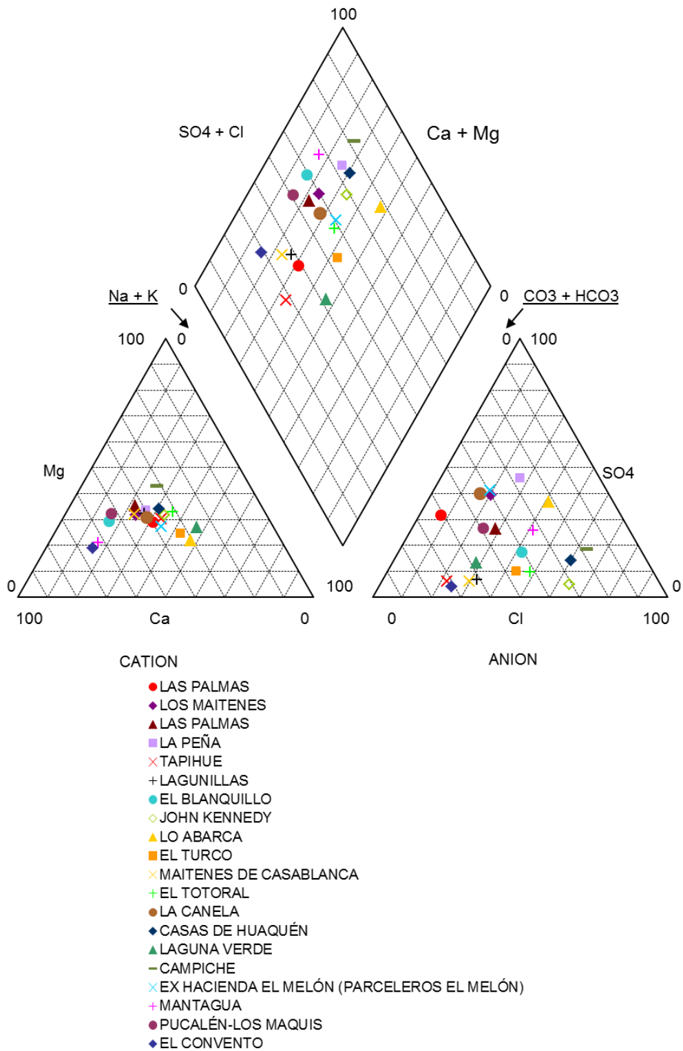
Figura 21: Representación mediante diagrama de Piper de las características químicas de las aguas subterráneas muestreadas en el sector de los acuíferos costeros. Se puede clasificar entre bicarbonatada o sulfatada cálcica y/o clorurada o sódica. Lo que indicaría procesos que ocurren en rocas carbonatadas o cristalinas, procesos de reducción de yeso u oxidación de sulfatos e influencia de aguas marinas.
