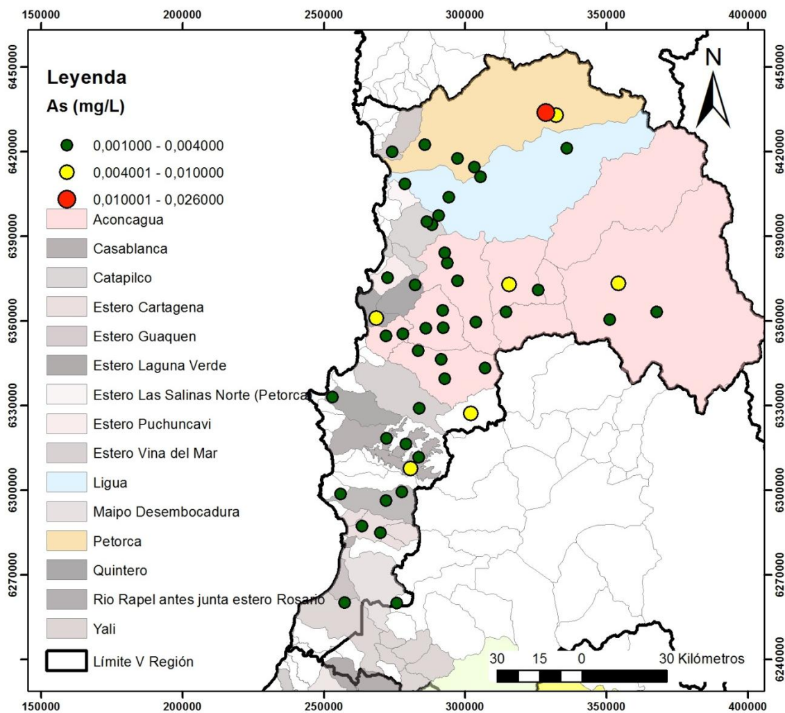
Figura 29: Concentraciones de arsénico por rango detectadas en los pozos muestreados en la V región.
