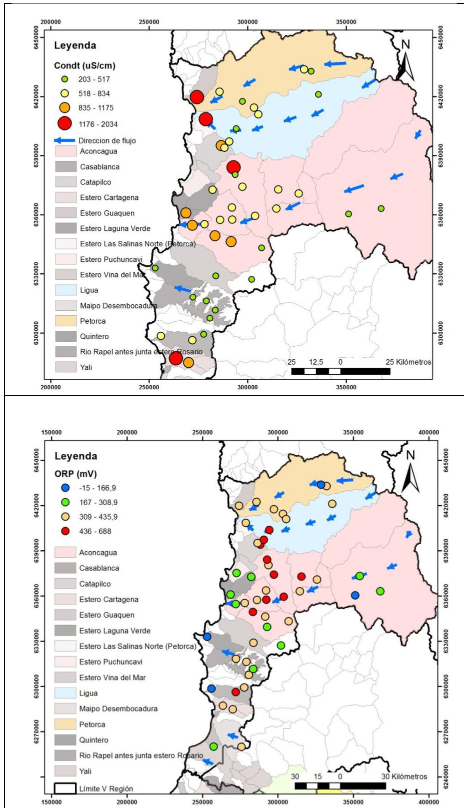
Figura 15: Parámetros físico químicos registrados in-situ en aguas de 49 pozos de la V Región. Arriba: datos de conductividad; Abajo: datos de potencial de óxido reducción. (Único valor negativo APR Valle los Olmos (acuífero de Petorca) ORP= -15 mV)
