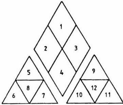
Figura 7: Clasificación de los diversos tipos de agua según diagrama de Piper.
