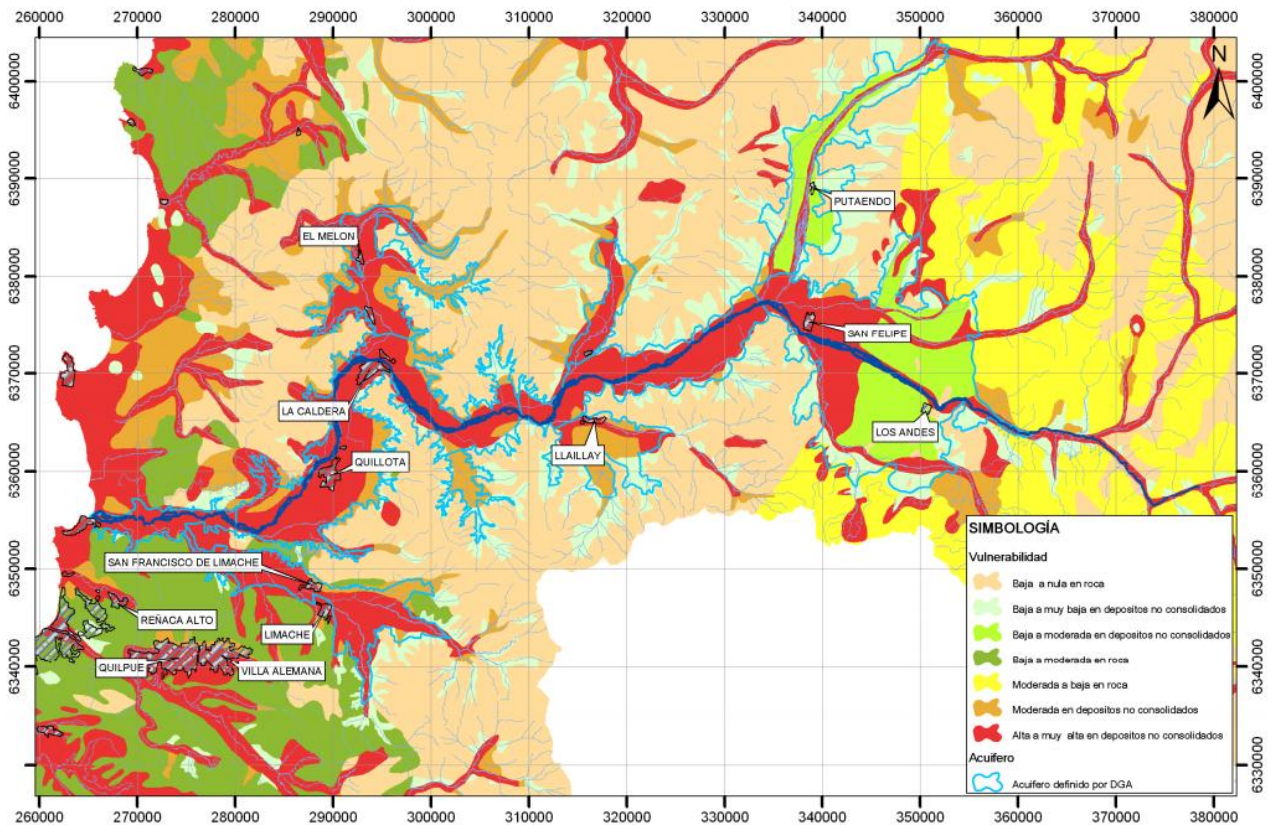
Figura 4: Mapa de vulnerabilidad de sector acuífero de Aconcagua. Fuente: Diagnóstico y Clasificación de Acuíferos, DGA 2009.
