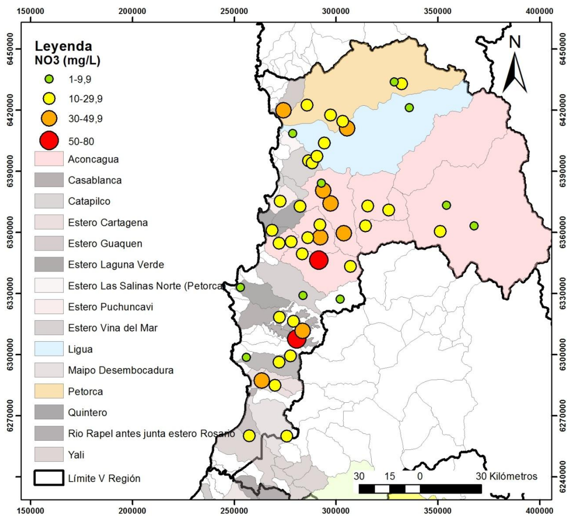
Figura 24: Representación de rangos de concentración de nitrato (NO 3 ) detectado en los pozos muestreados en acuíferos de la V Región.
