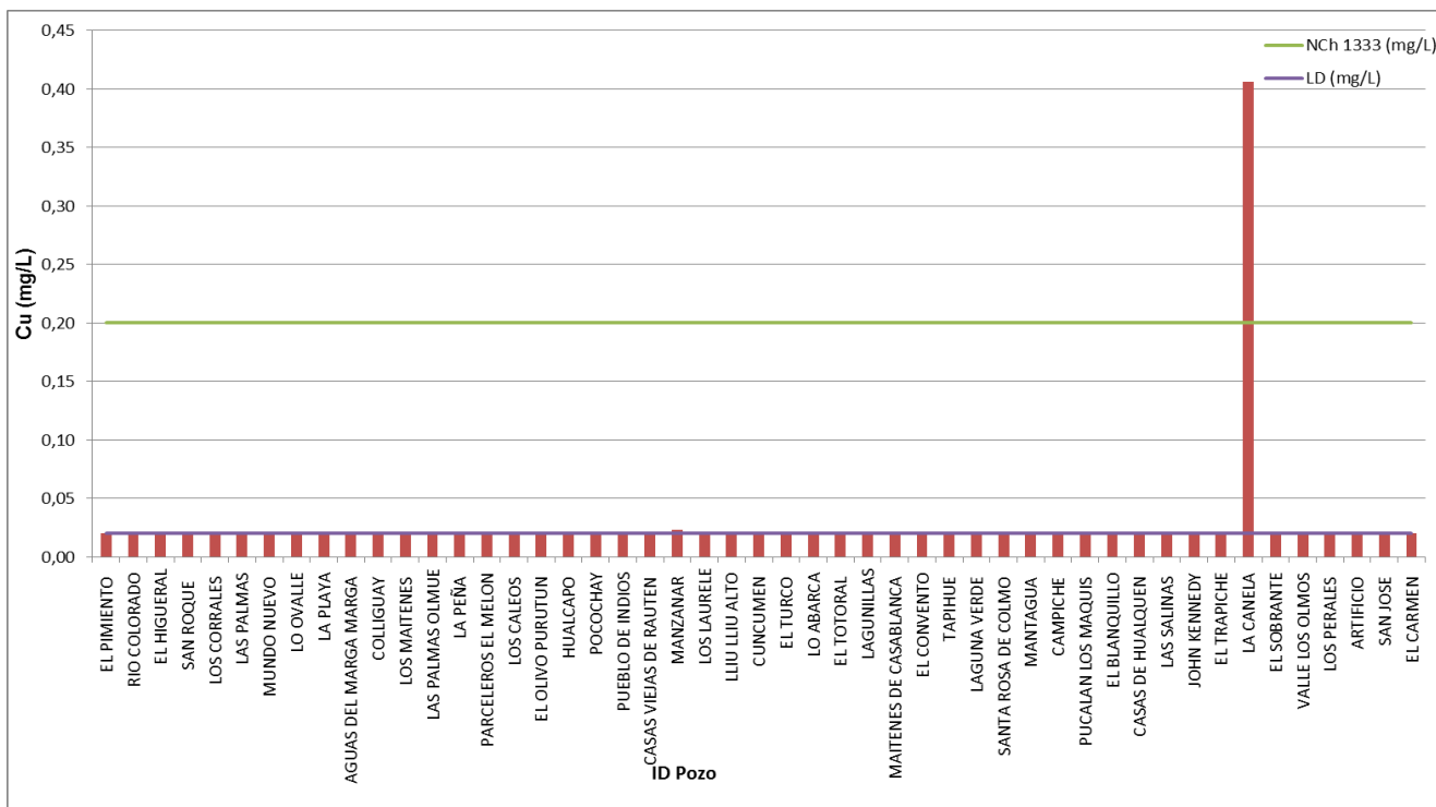
Figura 26: Concentración total de Cobre detectada en aguas subterráneas, comparada con límites establecidos en la norma de agua para riego (NCh 1333).
