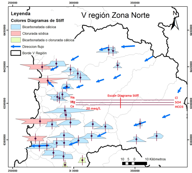
Figura 18: Detalle de Diagramas de Stiff en la zona norte de la V Región
