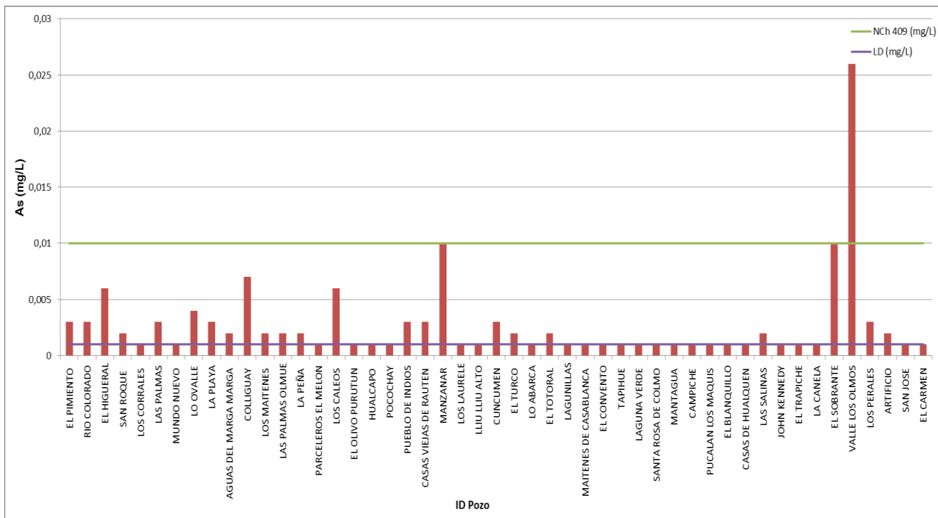
Figura 25: Concentración total de Arsénico detectada en aguas subterráneas, comparada con límites establecidos en la norma de agua potable (NCh 409).
