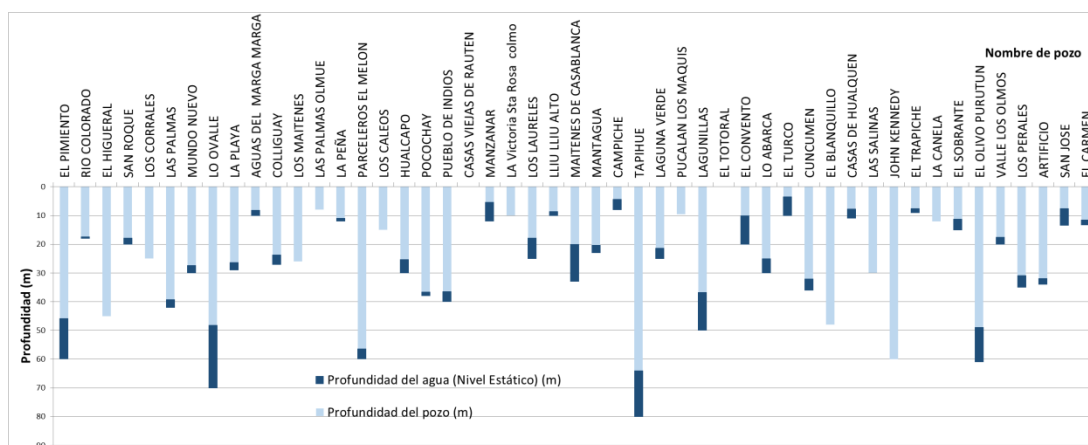
Figura 12: Profundidades de los pozos y sus respectivos registros de profundidad del agua medida en terreno (niveles estáticos)
