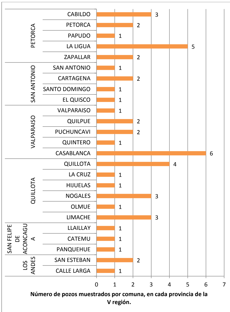
Figura 11: Distribución de puntos de muestreo en la V región.
