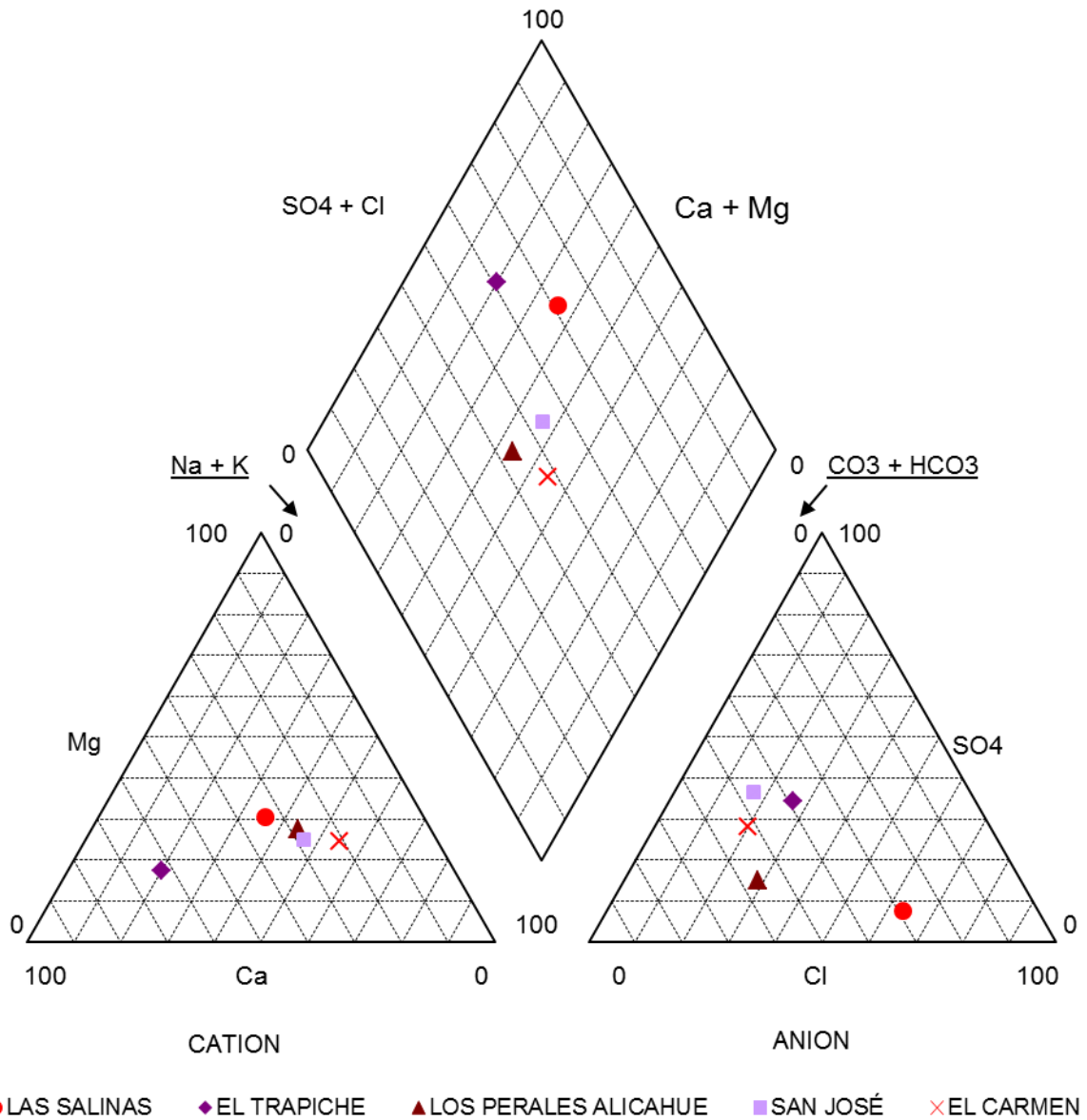
Figura 22: Representación mediante diagrama de Piper de las características químicas de las aguas subterráneas muestreadas en el acuífero La Ligua. Se puede clasificar como sulfatada o clorurada cálcica. Lo que indicaría procesos de reducción de yeso u oxidación de sulfatos con influencia de aguas marinas.
