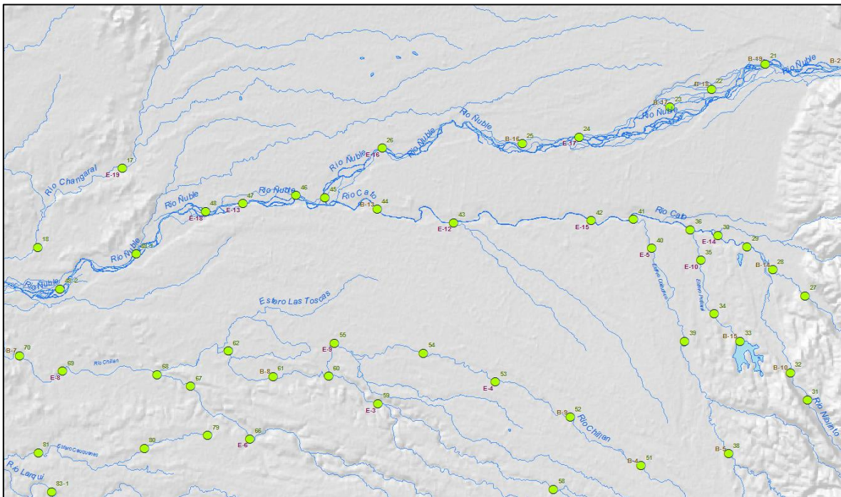
Figura 12. Topología (nudos) del modelo hidrológico.
