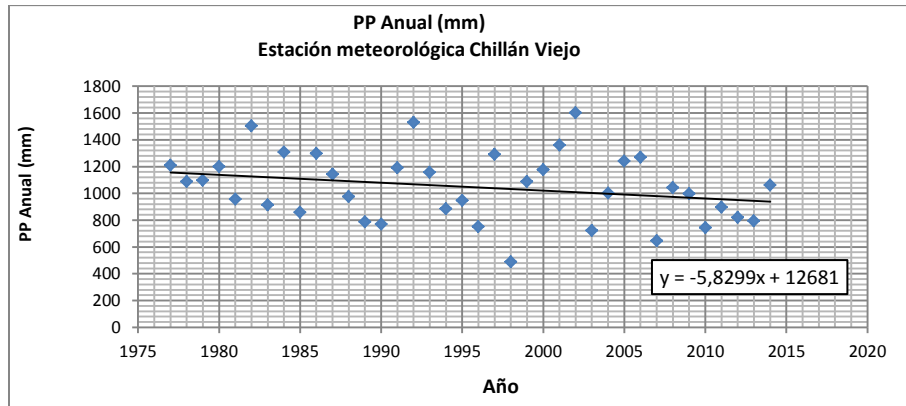
Figura 15. Precipitación anual. Estación meteorológica Chillán Viejo.
