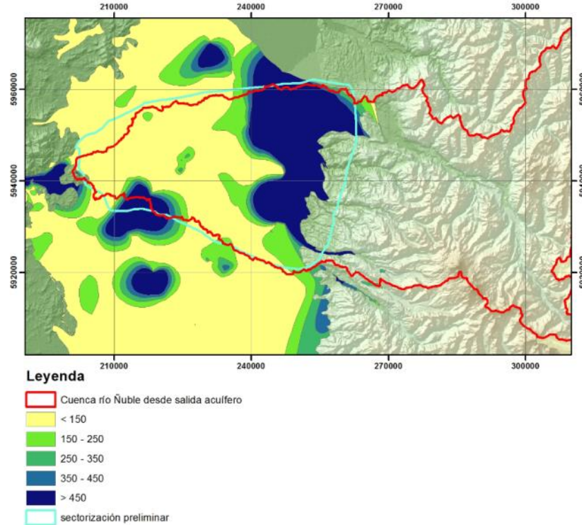
Figura 9. Transmisividad sector acuífero Ñuble Bajo.
