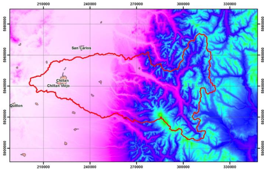
Figura 2. Modelo de Elevación Digital y delimitación cuenca del río Ñuble a partir de la confluencia con el río Chillán.
