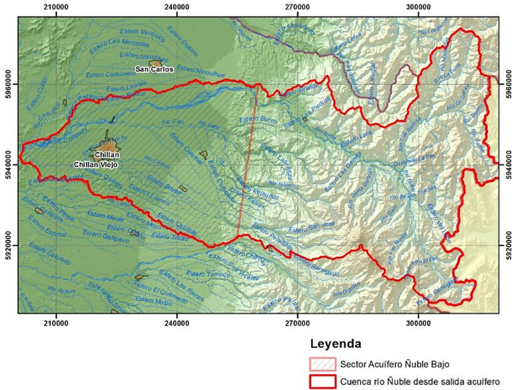
Figura 14. Propuesta de Sectorización. Ñuble Bajo.
