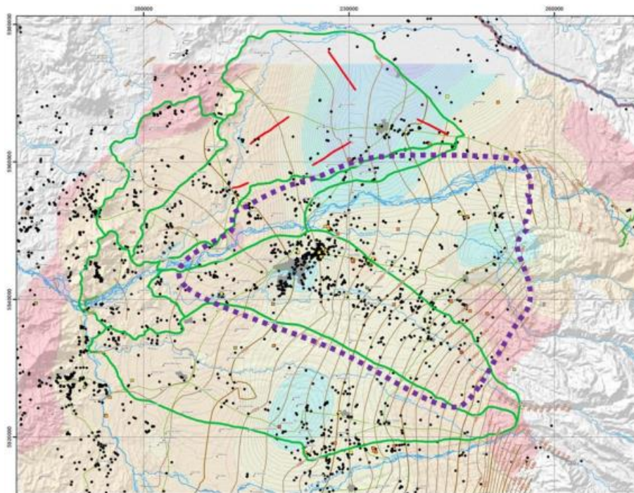
Figura 4. Sectorización preliminar en base a subcuencas, equipotenciales, ubicación de captaciones subterráneas, etc.
