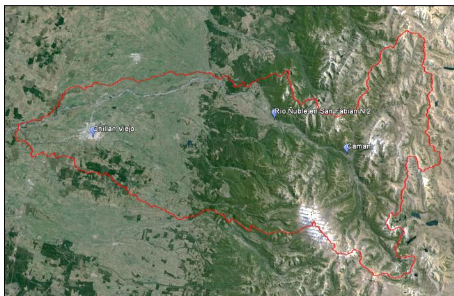
Figura 13. Estaciones meteorológicas empleadas en la estimación de la precipitación media anual característica de la cuenca aportante.
