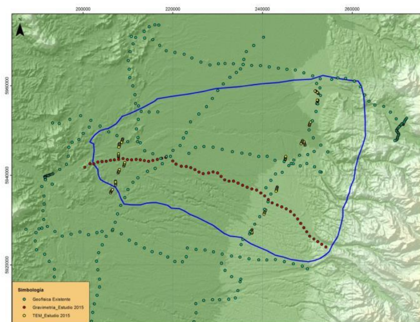
Figura 5. Geofísica existente en la zona de estudio. En verde: gravimetría DGA/Aquaterra (2011). En rojo: gravimetría DGA/Subterránea SpA (2015). En amarillo: TEM DGA/Subterránea (2015).
