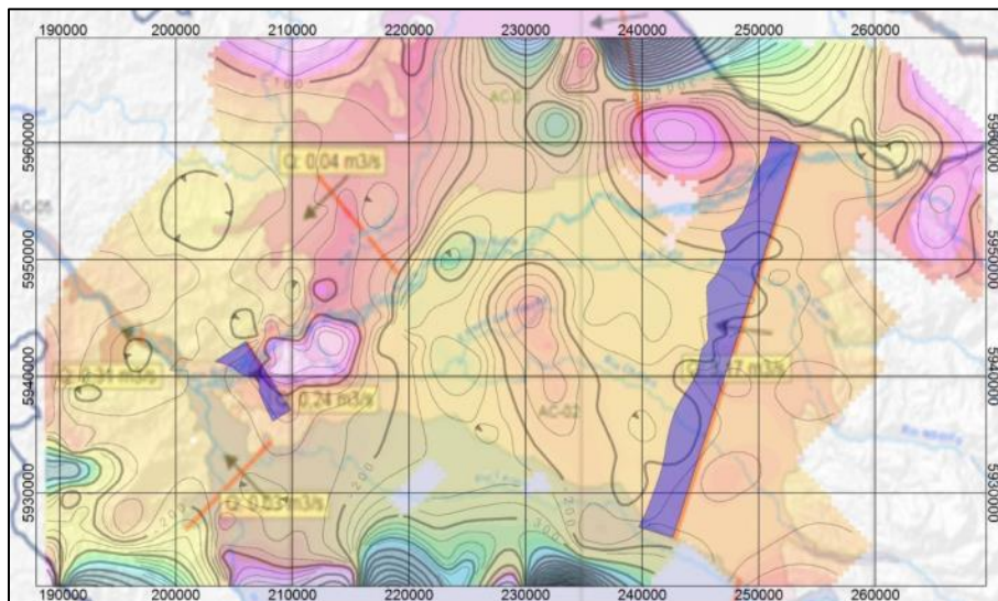
Figura 6. Profundidad de basamento y secciones de entrada y salida (sector acuífero Ñuble Bajo).
