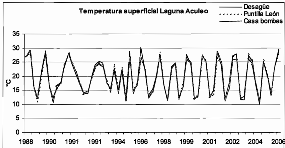
Figura 3. Temperatura superficial de la laguna (Primavera 1988-Verano 2006) en las tres estaciones de monitoreo.
