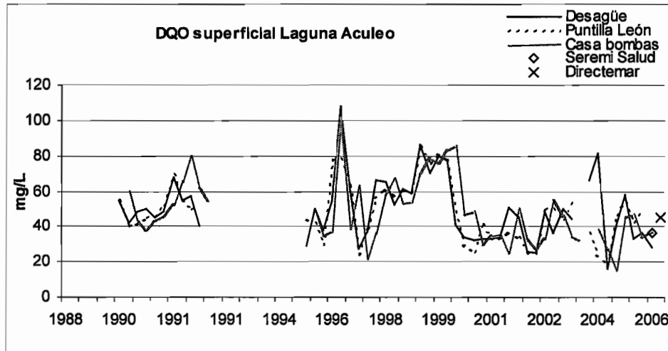
Figura 7. Demanda Química de Oxígeno (DQO) superficial de la laguna (Primavera 1988-Verano 2006) en las tres estaciones de monitoreo.
