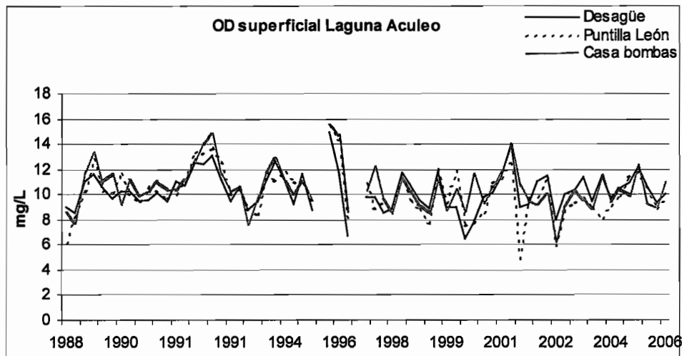
Figura 6. Oxígeno Disuelto (OD) superficial de la laguna (Primavera 1988-Verano 2006) en las tres estaciones de monitoreo.
