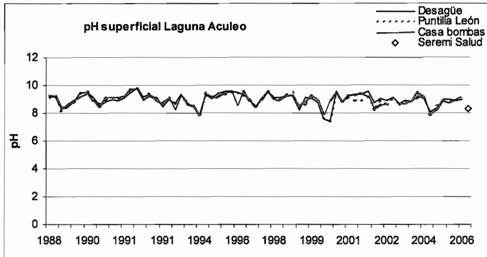
Figura 5. pH de la laguna (Primavera 1988-Verano 2006) en las tres estaciones de monitoreo.
