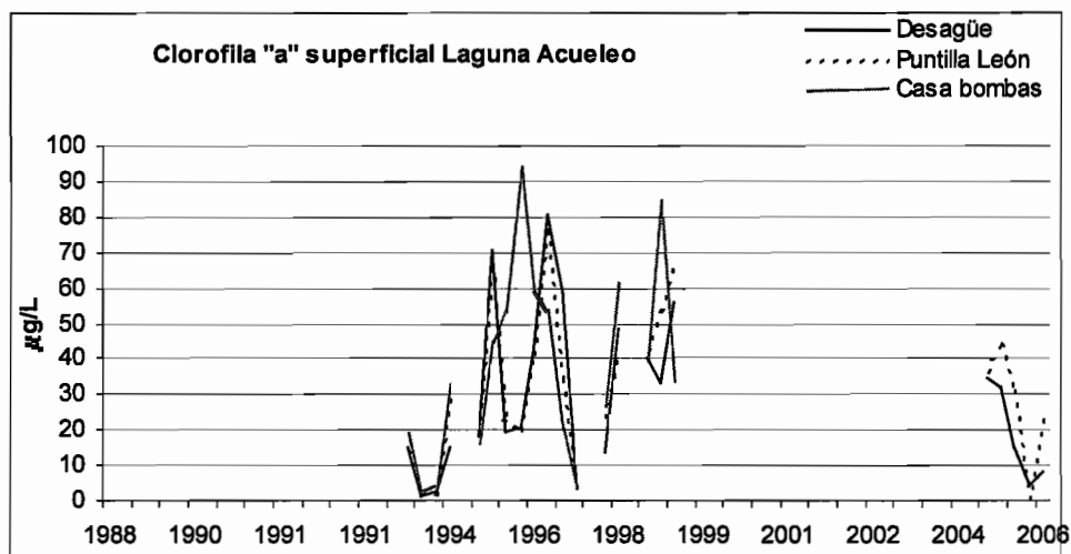
Figura 10. Clorofila "a" superficial de la laguna (Primavera 1988-Verano 2006) en las tres estaciones de monitoreo.
