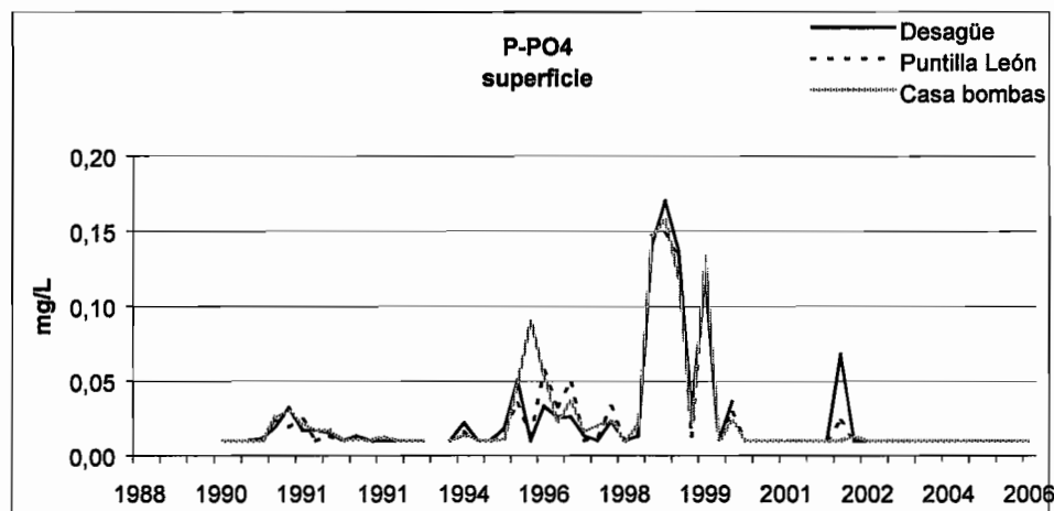
Figura 9. Fósforo disponible superficial de la laguna (Primavera 1988-Verano 2006) en las tres estaciones de monitoreo.
