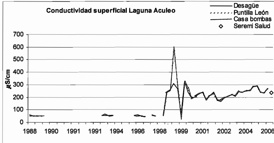
Figura 4. Conductividad eléctrica de la laguna (Primavera 1988-Verano 2006) en las tres estaciones de monitoreo.
