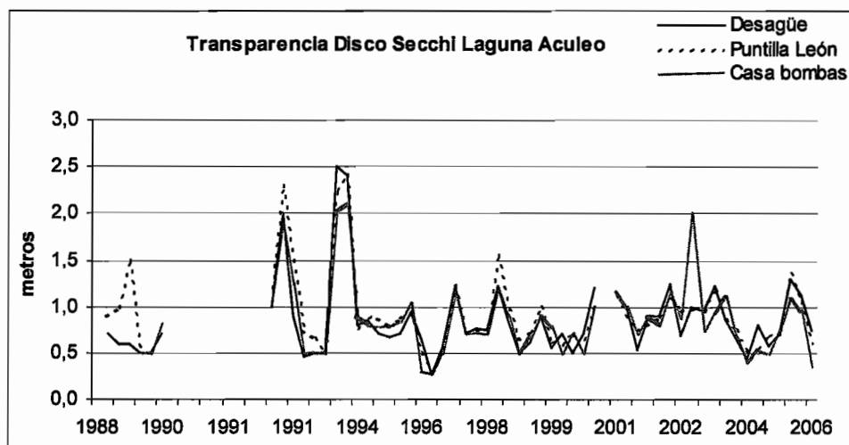
Figura 2. Transparencia Disco Secchi de la laguna (Primavera 1988-Verano 2006) en las tres estaciones de monitoreo.
