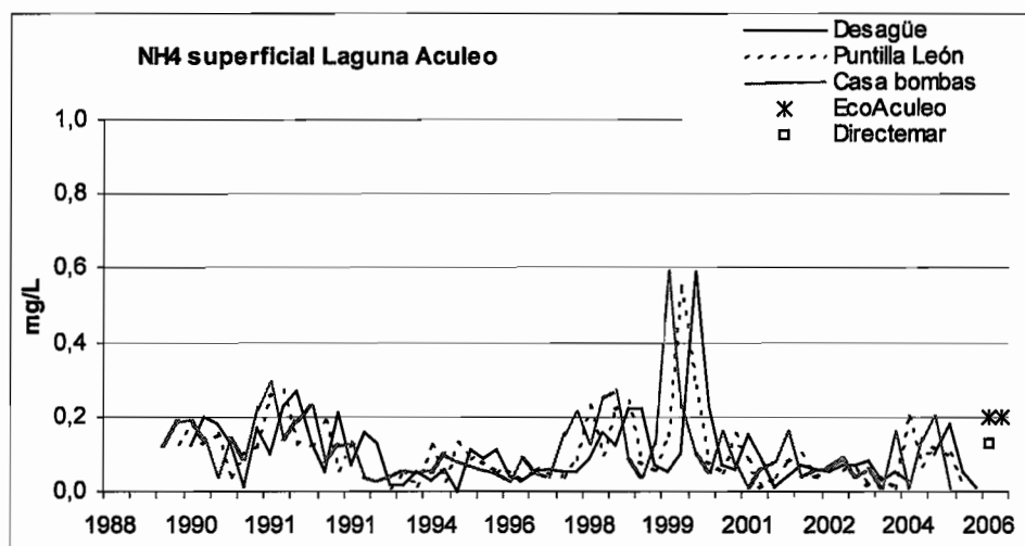
Figura 9. Nitrógeno amoniacal superficial de la laguna (Primavera 1988-Verano 2006) en las tres estaciones de monitoreo.
