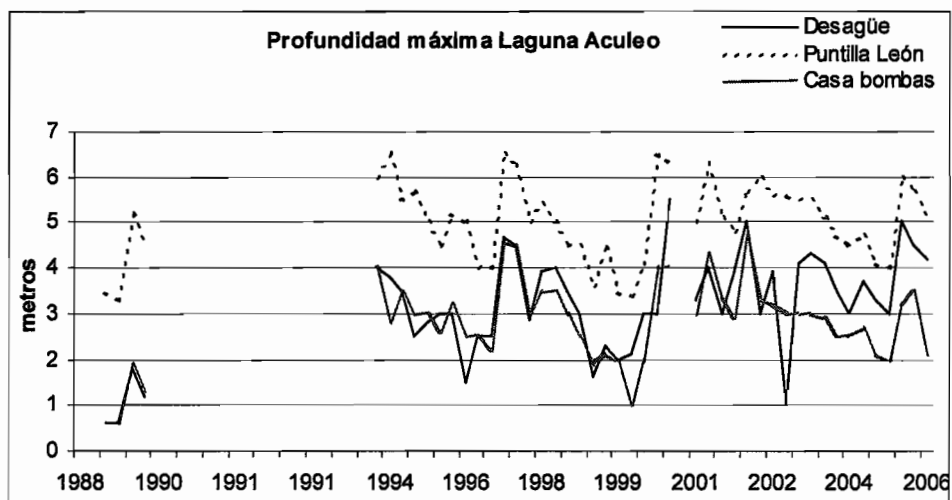
Figura 1. Profundidad máxima de la laguna (Primavera 1988-Verano 2006) en las tres estaciones de monitoreo.
