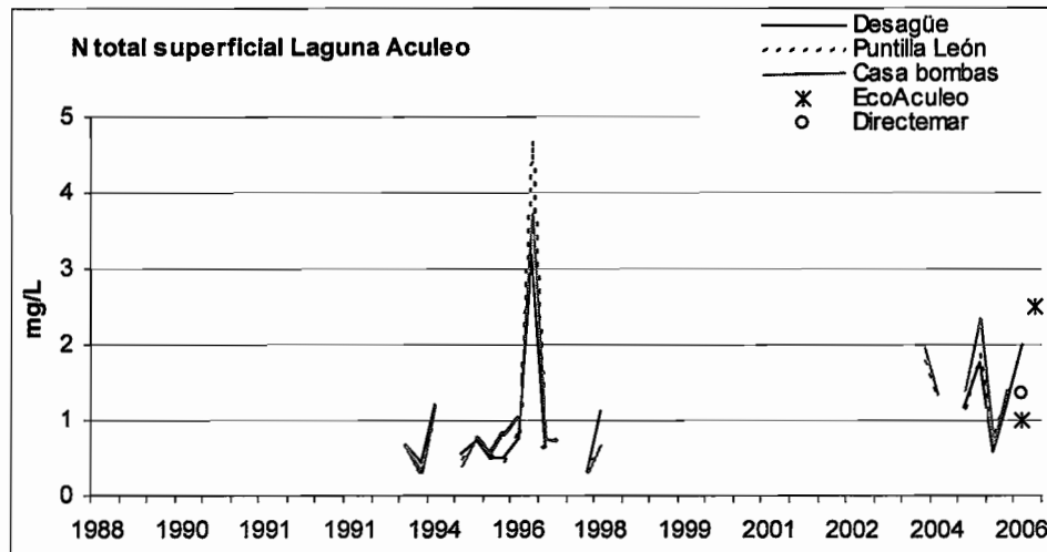
Figura 8. Nitrógeno Total superficial de la laguna (Primavera 1988-Verano 2006) en las tres estaciones de monitoreo.
