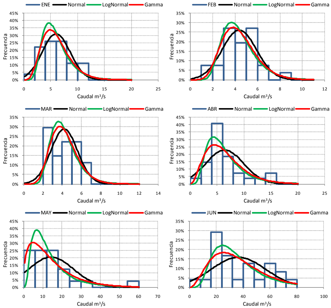
Figura 16. Ajuste Distribución Probabilística Caudales Mensuales Meses Enero-Junio. Estación RIO IÑAQUE EN MAFIL.
