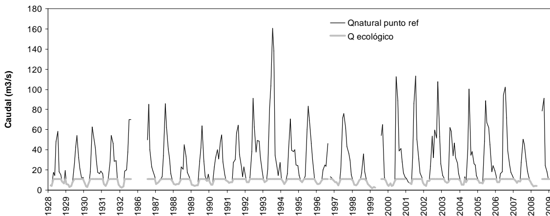
Figura 21. Serie de caudales mensuales en el punto de referencia y serie de caudal ecológico en el mismo punto, calculado como el 40% del caudal medio anual por mes.
