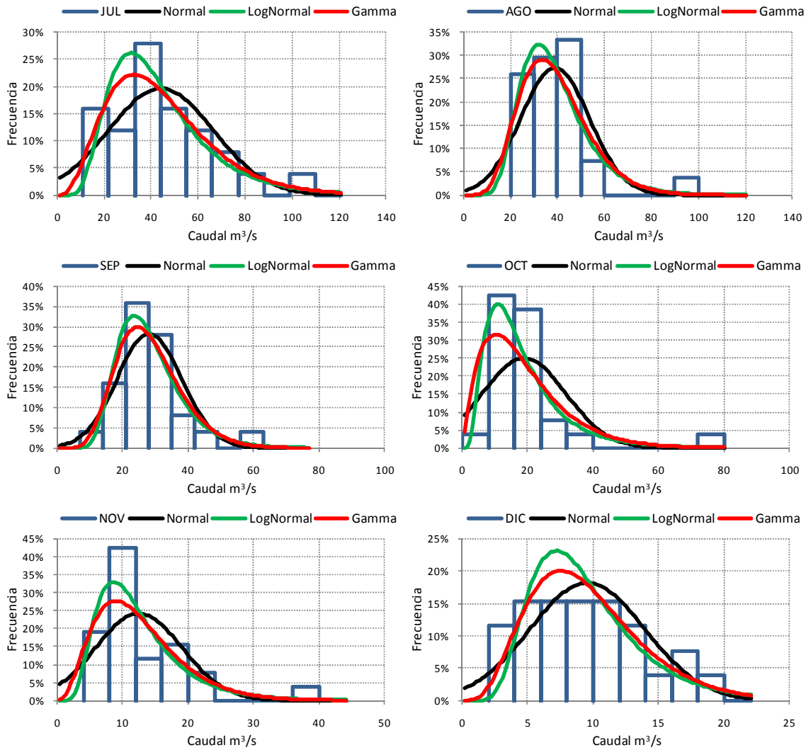
Figura 17. Ajuste Distribución Probabilística Caudales Mensuales Meses Julio-Diciembre. Estación RIO IÑAQUE EN MAFIL.
