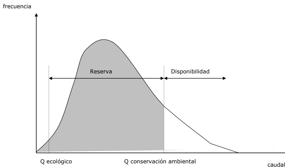
Figura 23. Procedimiento para definir reserva (incluyendo caudal ecológico) para conservación ambiental y disponibilidad.
