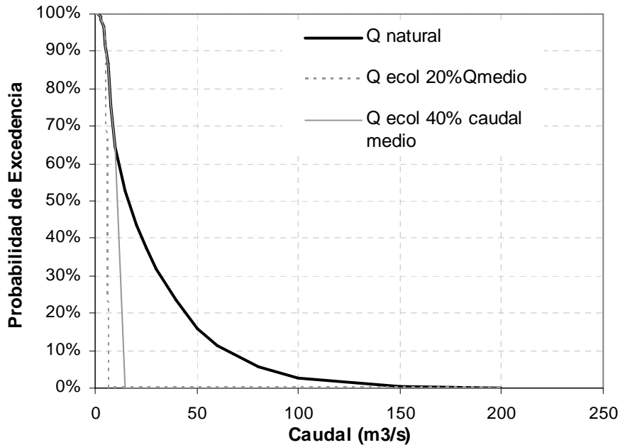
Figura 22. Probabilidad de excedencia de caudal para las series del río, y del caudal ecológico en el punto de referencia.
