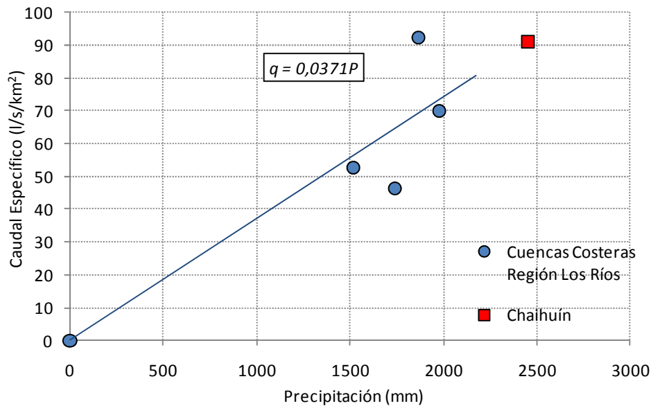
Figura 14. Estimación Caudal Específico Chaihuín.
