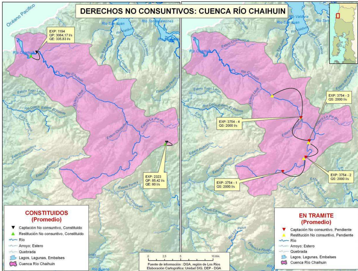
Figura 10. Situación de Derechos No Consuntivos constituidos y en trámite en la cuenca del río Chaihuín.
