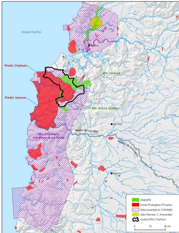
Figura 4: Áreas protegidas cuenca río Chaihuín.
