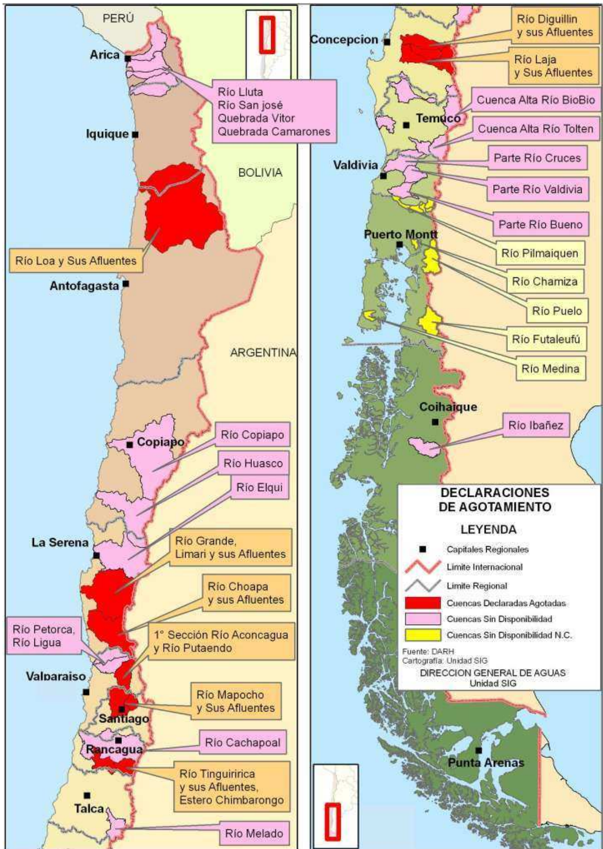
Figura 2. Ríos sin disponibilidad y agotados en Chile.
