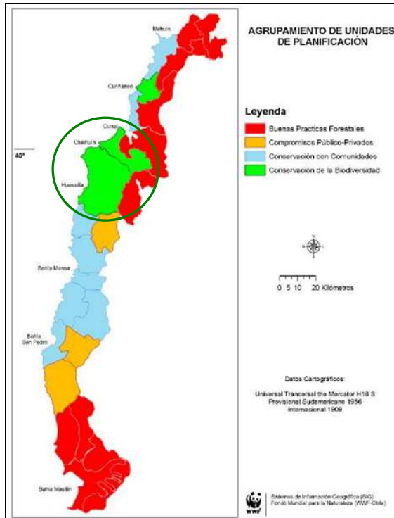
Figura 7: Unidades de planificación Cordillera de La Costa. Fuente Plissock, P. et al, 2005.
