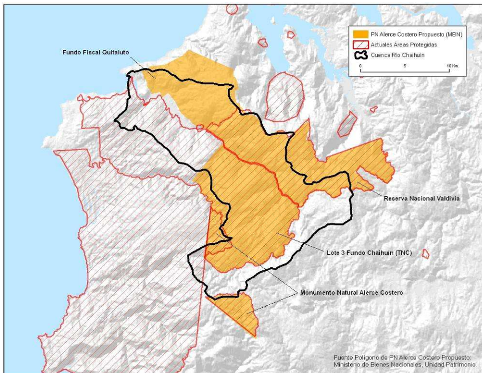
Figura 8: Tierras que conformarán el Parque Nacional Alerce Costero.
