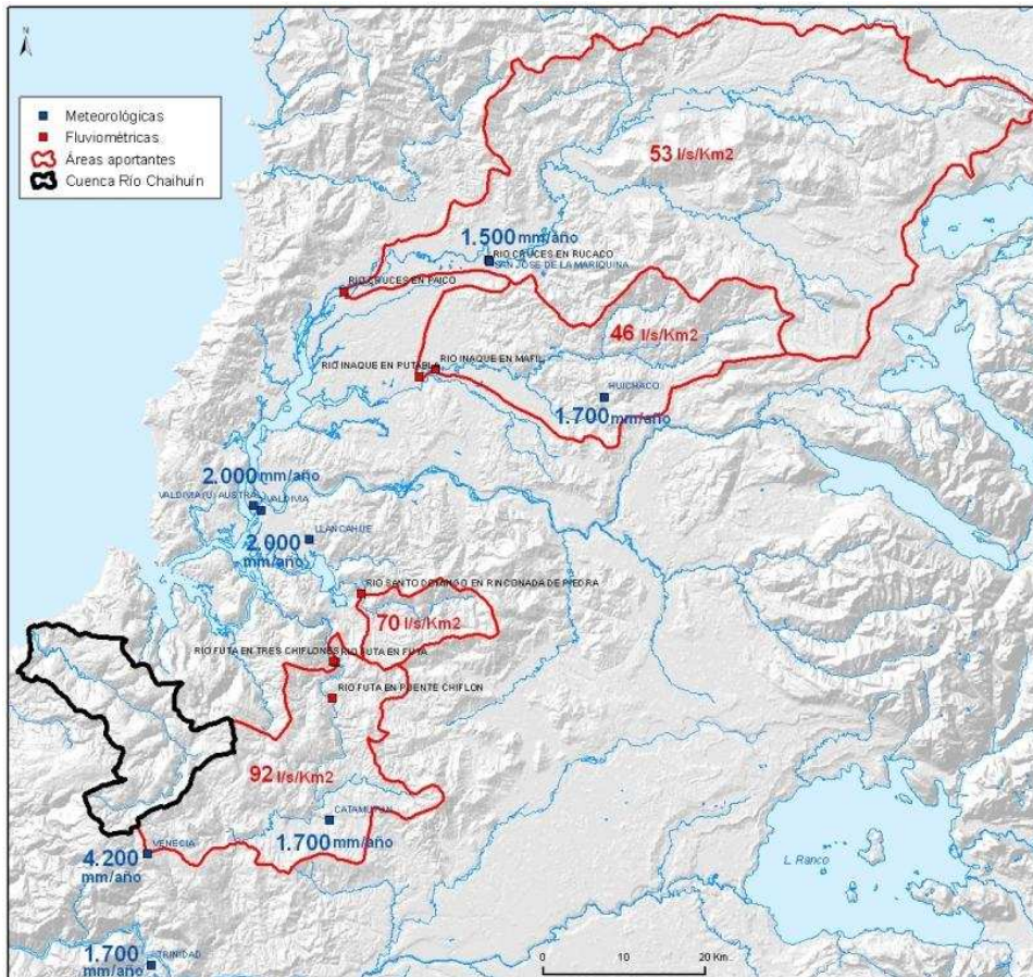
Figura 12. Precipitación Media Anual y Rendimiento Medio Observado.
