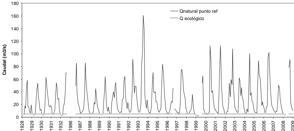
Figura 20. Serie de caudales mensuales en el punto de referencia y serie de caudal ecológico en el mismo punto, calculado como el 20% del caudal medio anual por mes.
