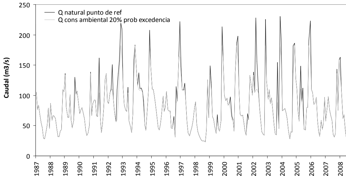
Figura 25. Serie de caudales mensuales en el punto de referencia y serie de caudal de conservación ambiental en el mismo punto, calculado como el valor mensual de probabilidad de excedencia 20%.
