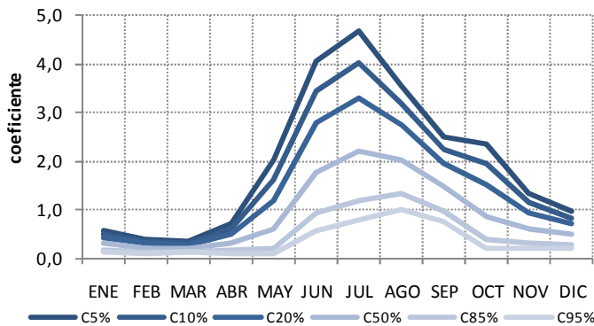
Figura 18. Coeficientes Mensuales de Frecuencia. Río Iñaque en Máfil.
