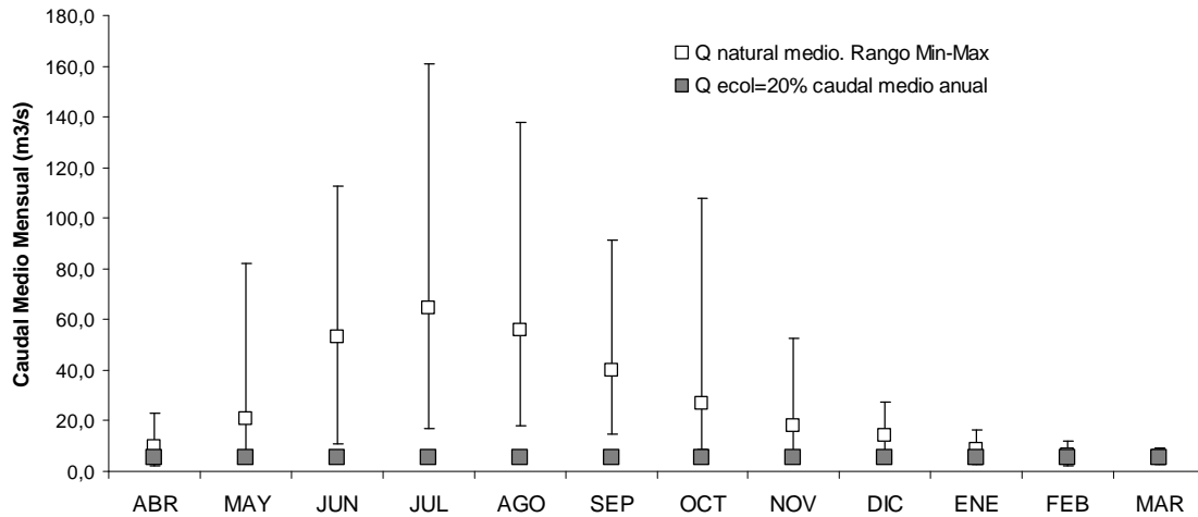
Figura 19. Valores medios mensuales y rango mínimo y máximo de la serie de caudales mensuales en el punto de referencia.
