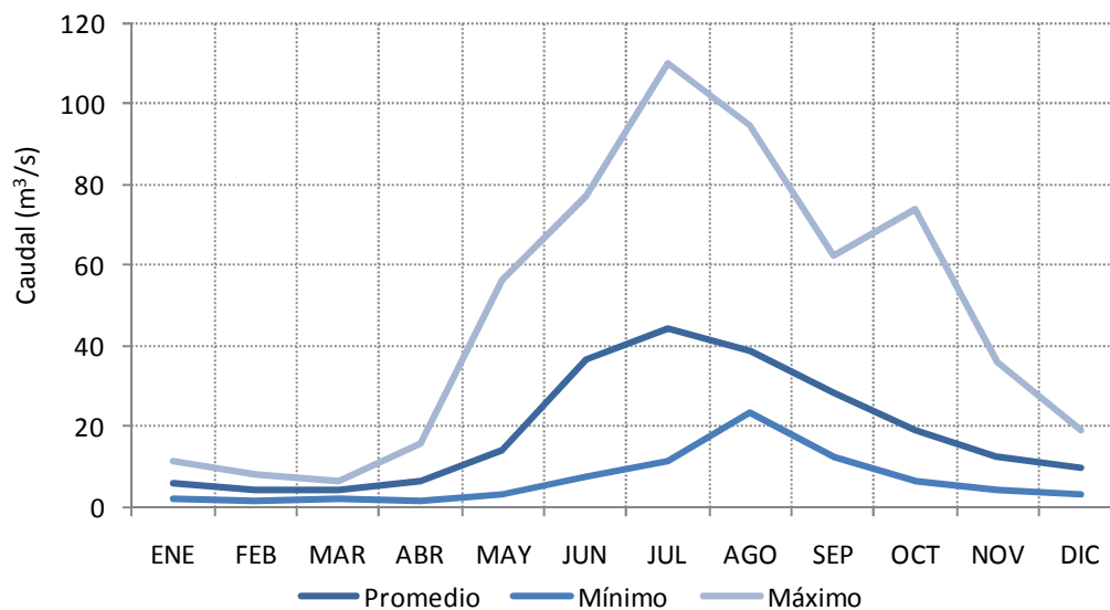
Figura 15. Caudales Mensuales Río Iñaque en Máfil. Promedio, Mínimo y Máximo.
