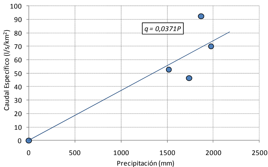
Figura 13. Relación Empírica Precipitación-Caudal Específico. Cuencas Costeras Región de Los Ríos.
