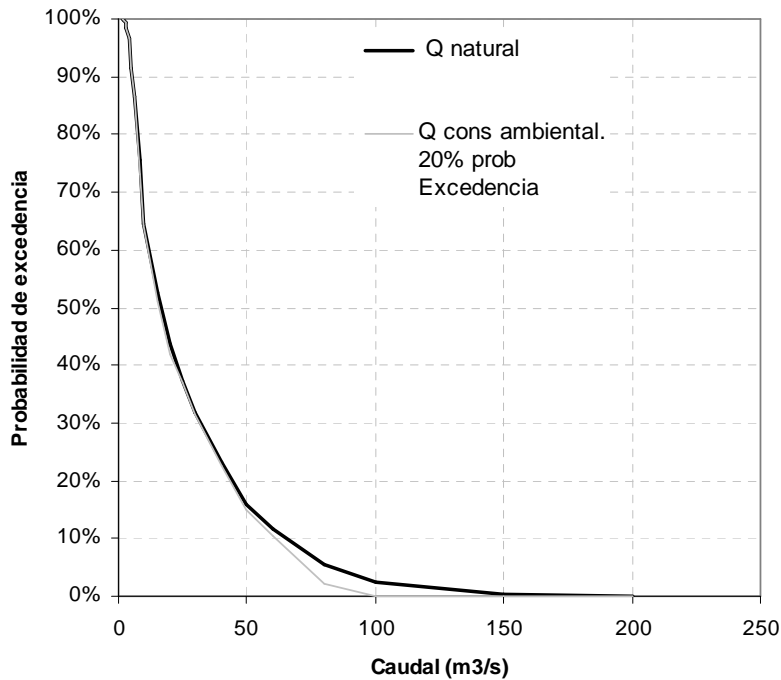
Figura 24. Distribución de probabilidad del río Chaihuín en el punto de referencia en condiciones naturales y considerando un caudal de conservación ambiental equivalente al de 20% de probabilidad de excedencia en condiciones naturales.
