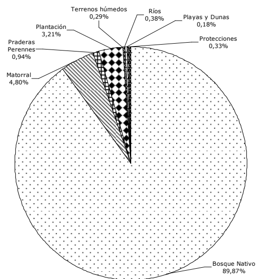
Figura 6: Usos de suelo cuenca río Chaihuín. Fuente: Catastro de Bosque Nativo, Conaf 2006.
