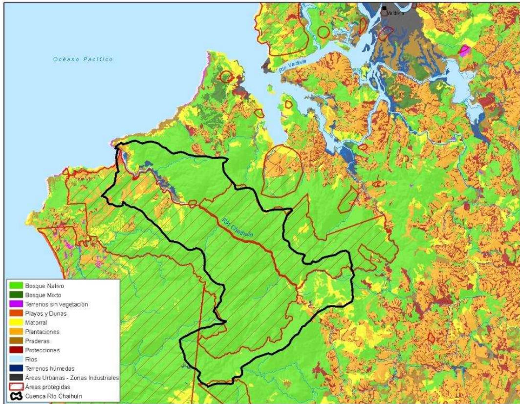
Figura 5: Usos de suelo cuenca río Chaihuín. Fuente: Catastro de Bosque Nativo, Conaf 2006.
