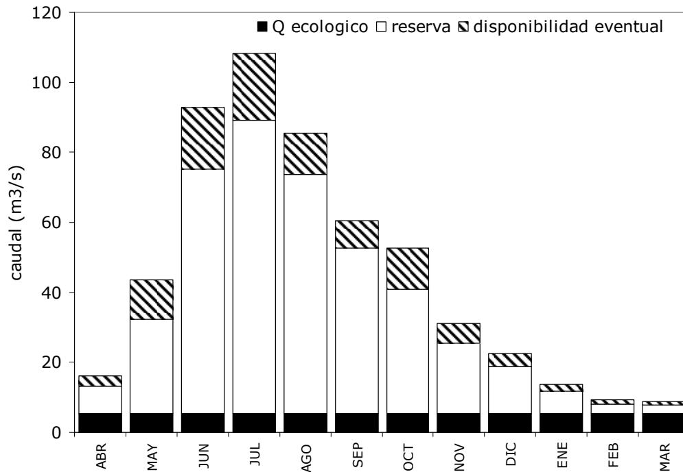
Figura 26. Caudal ecológico, de reserva y de disponibilidad eventual en el punto de referencia.
